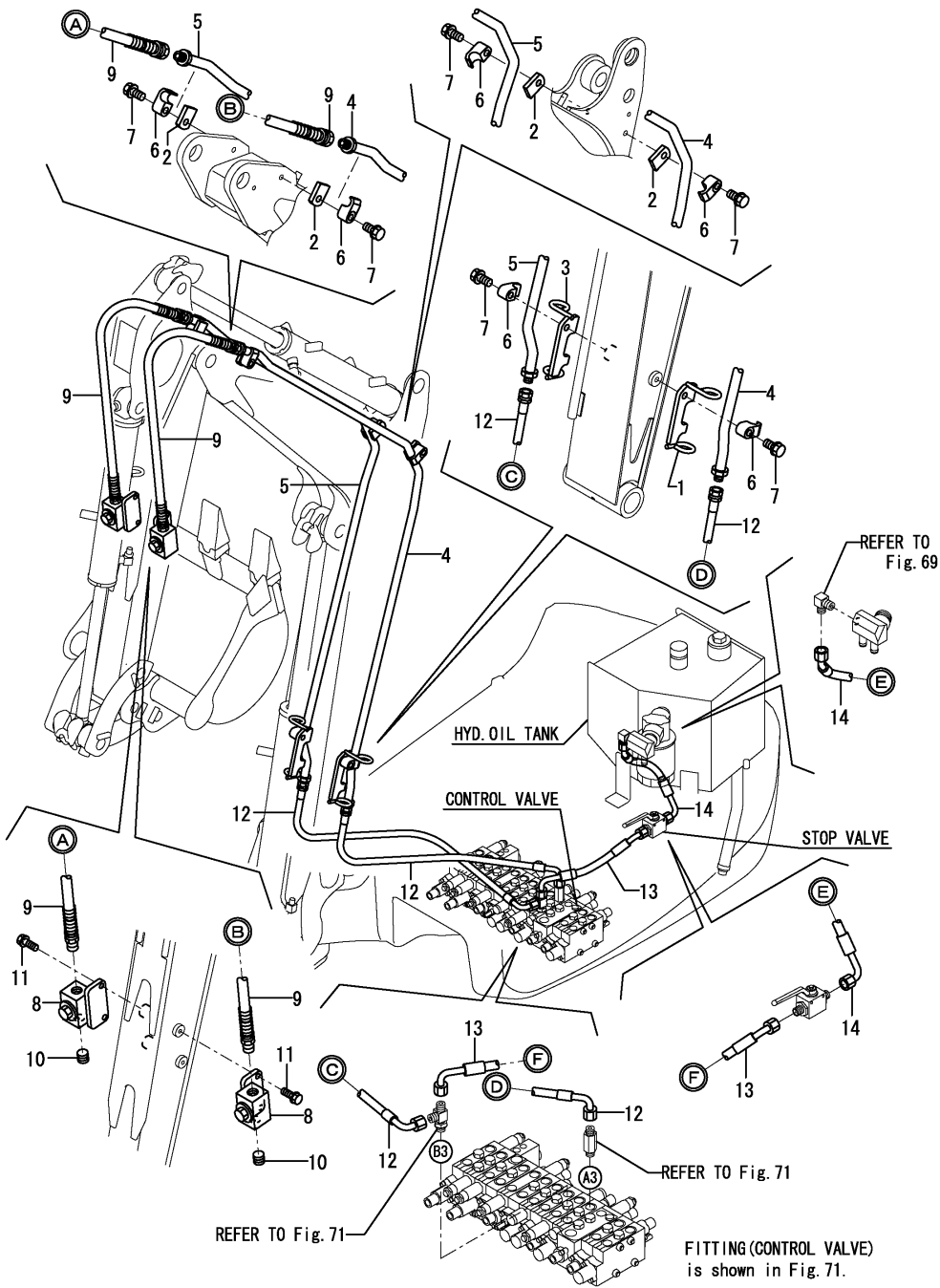
Fig.72. HYD.OIL PIPING(P.T.O.)
