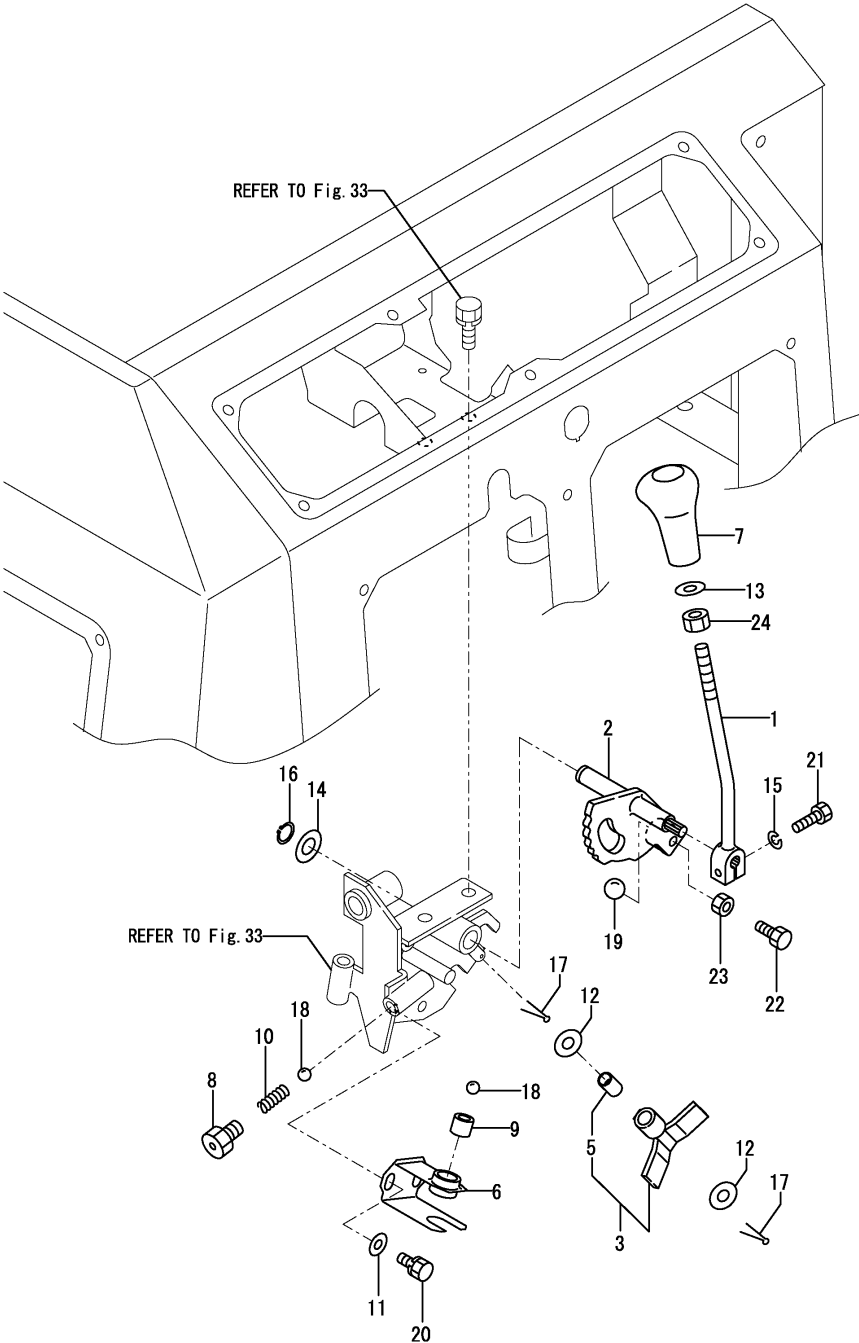
OCS10-G52500 Fig.25. FR LEVER
