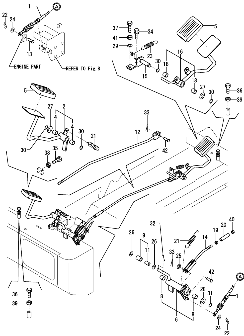
Fig.7. FOOT ACCELERTOR
