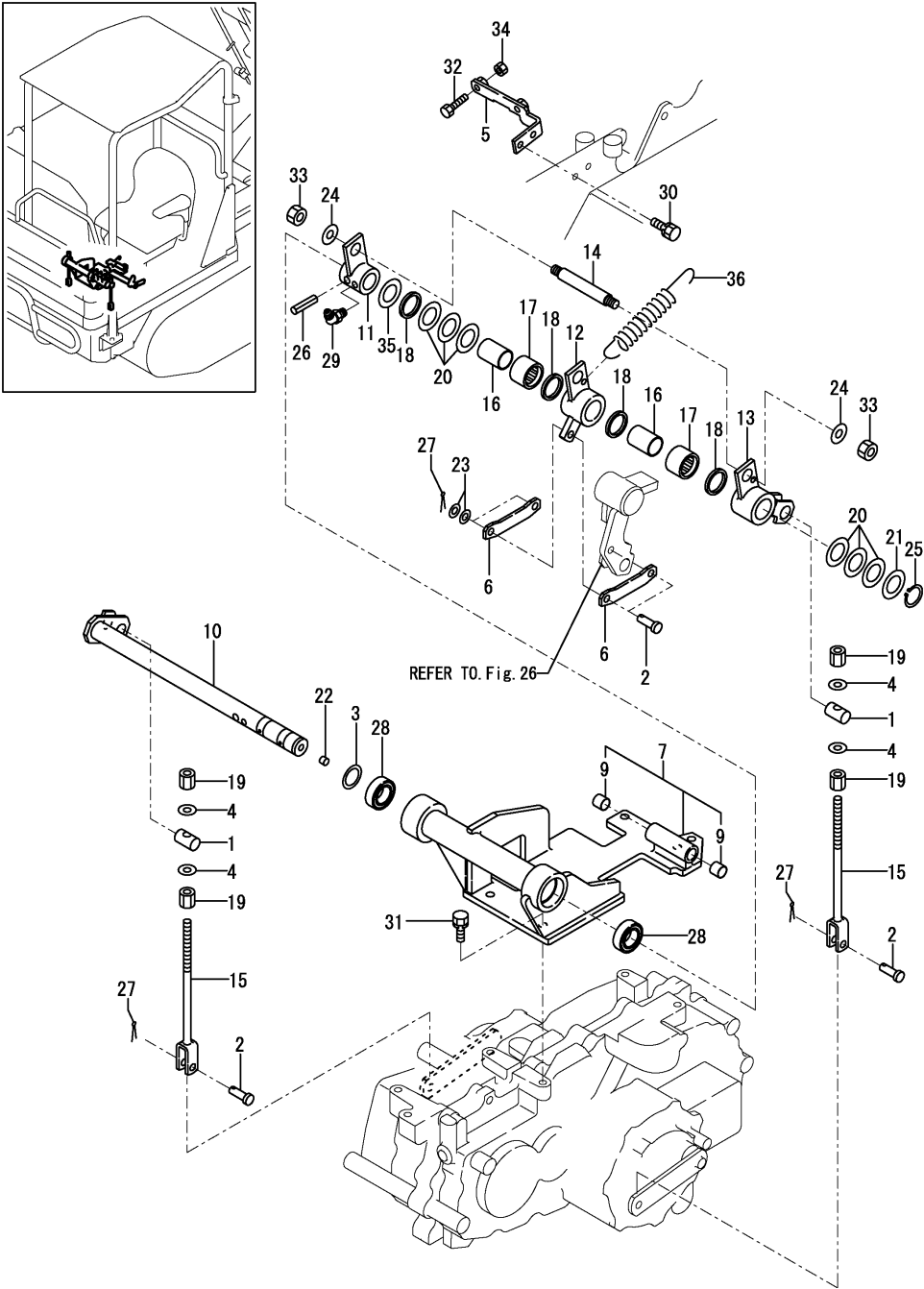
Fig.30. BRAKE(LINK)
