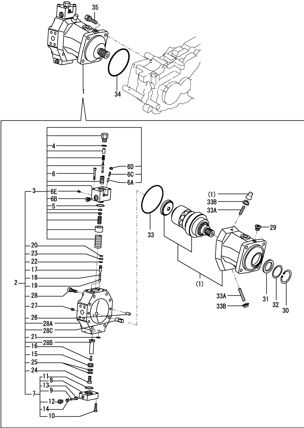
Fig.43. MOTOR
