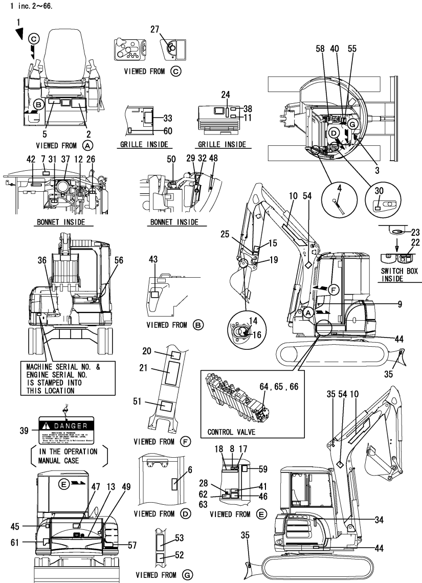
Fig.1. LABEL(CABIN)
