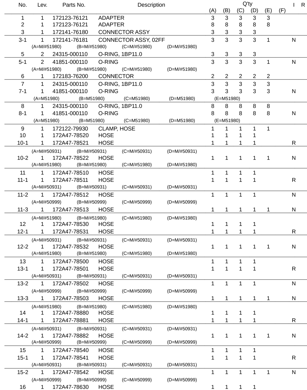
(A)=VIO55-5(US) (D)=VIO55-5(KR) (B)=VIO55-5(AS) (E)=VIO55-5(SG) (C)=VIO55-5(NZ) (F)=
