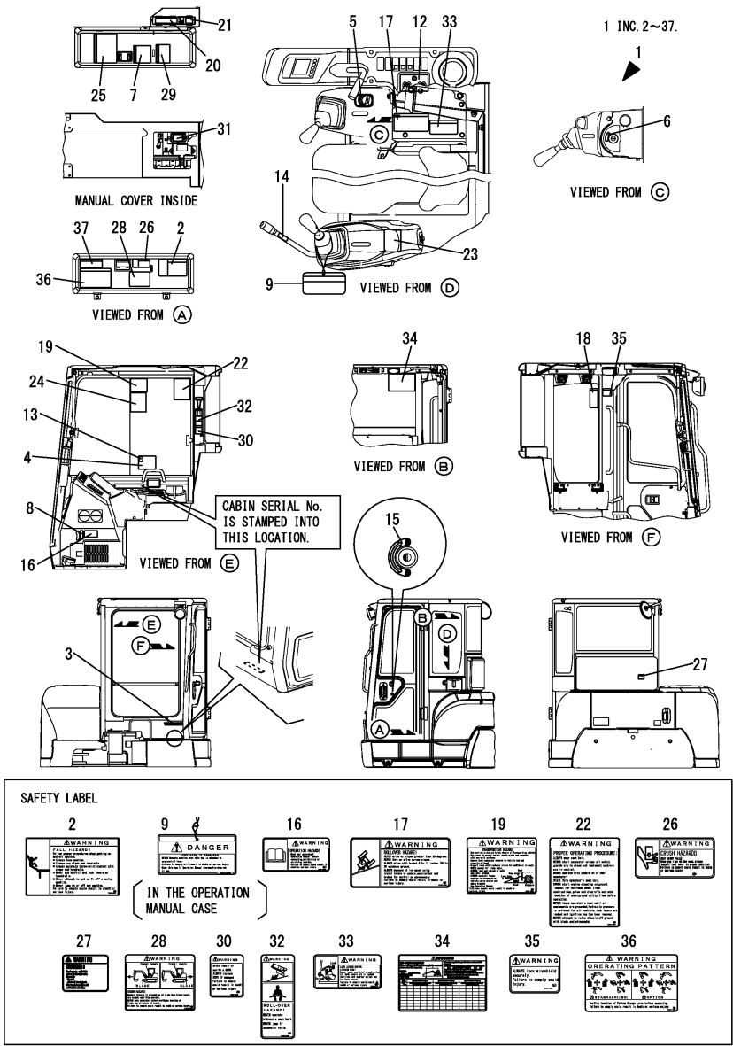
Fig.5. LABEL(CABIN)
