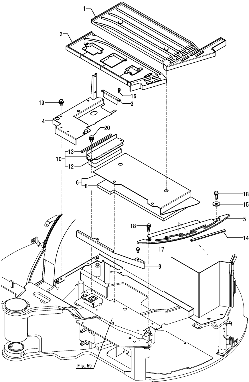
Fig.83. STEP(CABIN)
