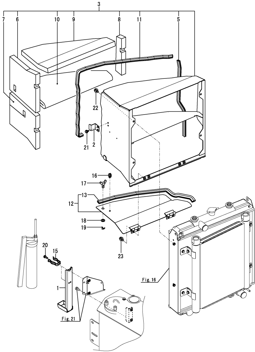
Fig.18. DUCT
