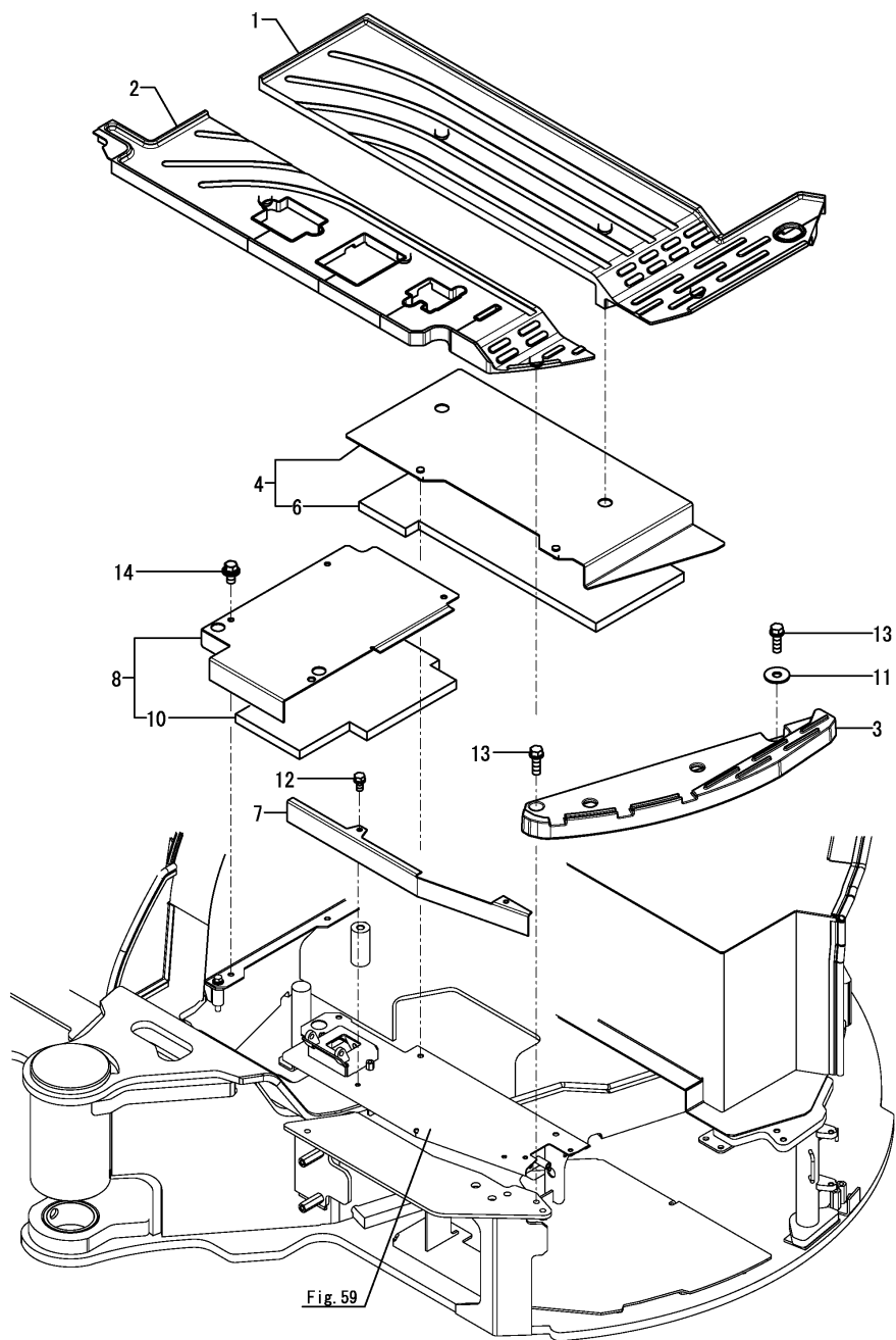
Fig.84. STEP(CANOPY)
