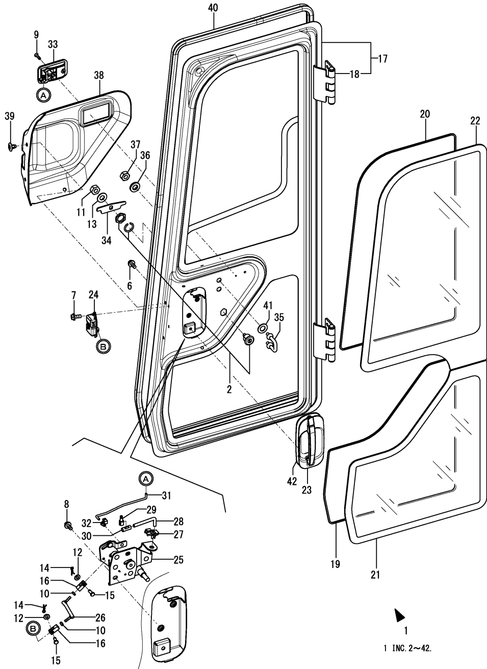
Fig.106. CABIN DOOR(2)
