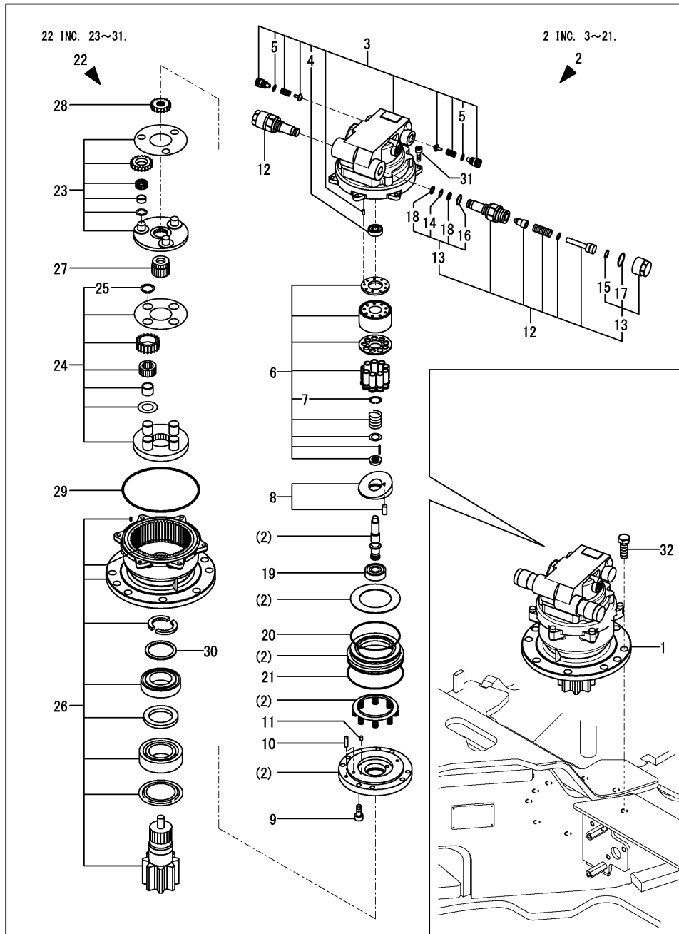
Fig.132. TURNING MOTOR
