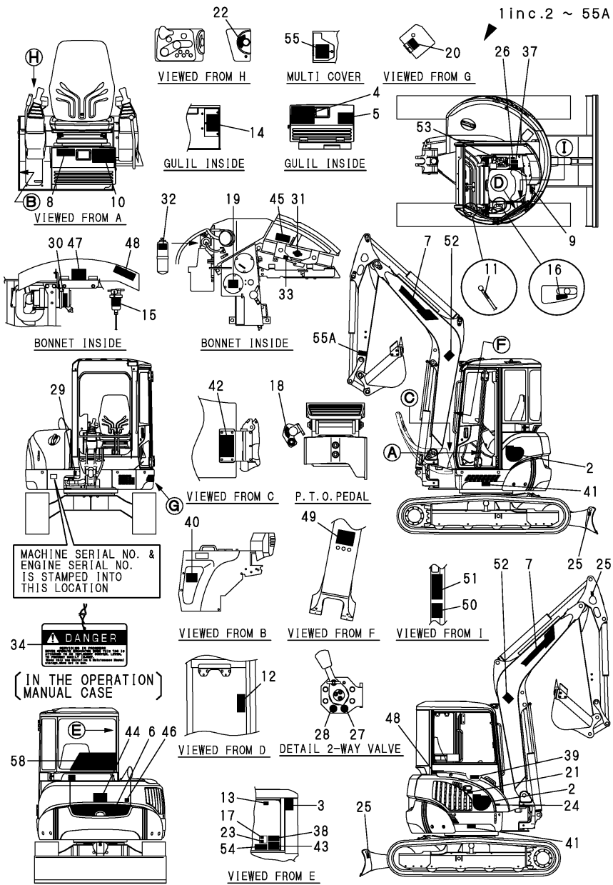
Fig.1. LABEL(CABIN)
