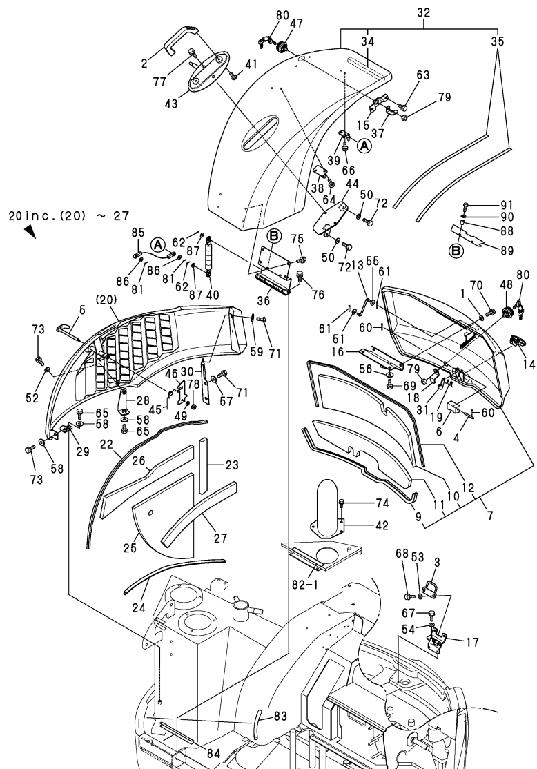
Fig.38. BONNET
