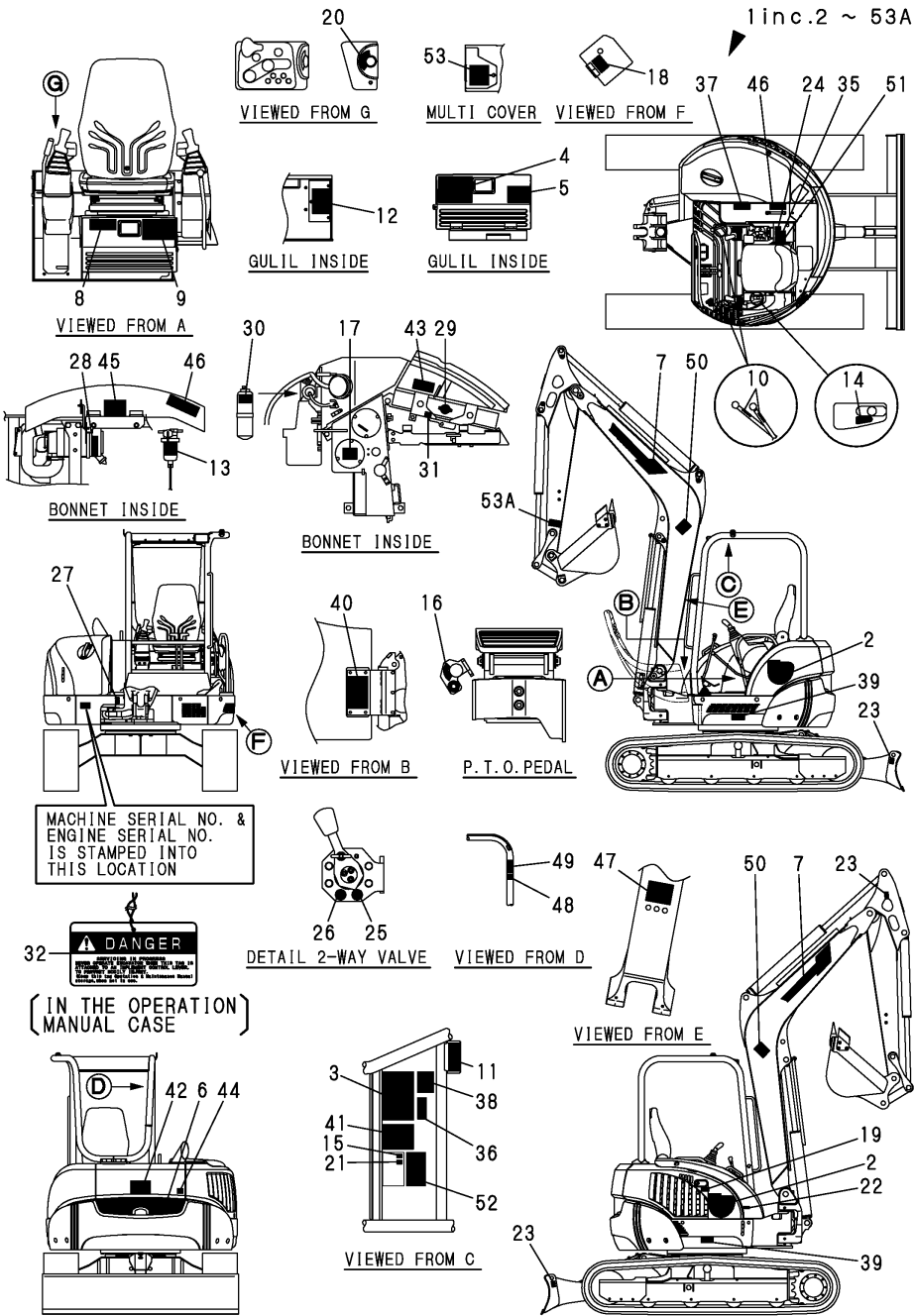
Fig.2. LABEL(CANOPY)
