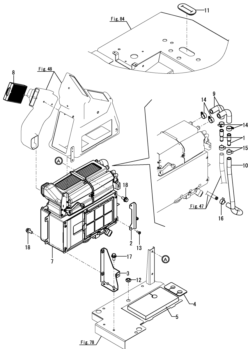
Fig.45. HEATER(UNIT)
