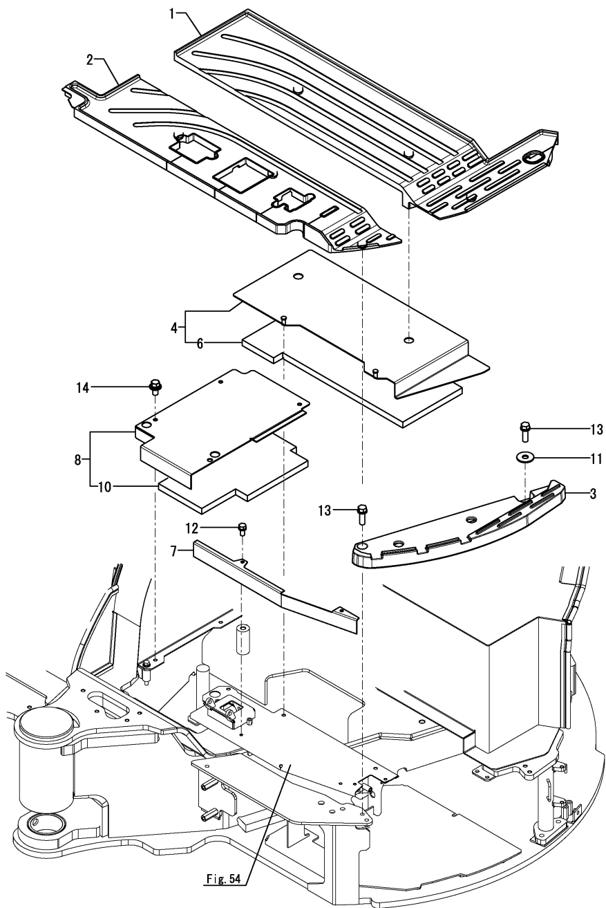
Fig.79. STEP(CANOPY)
