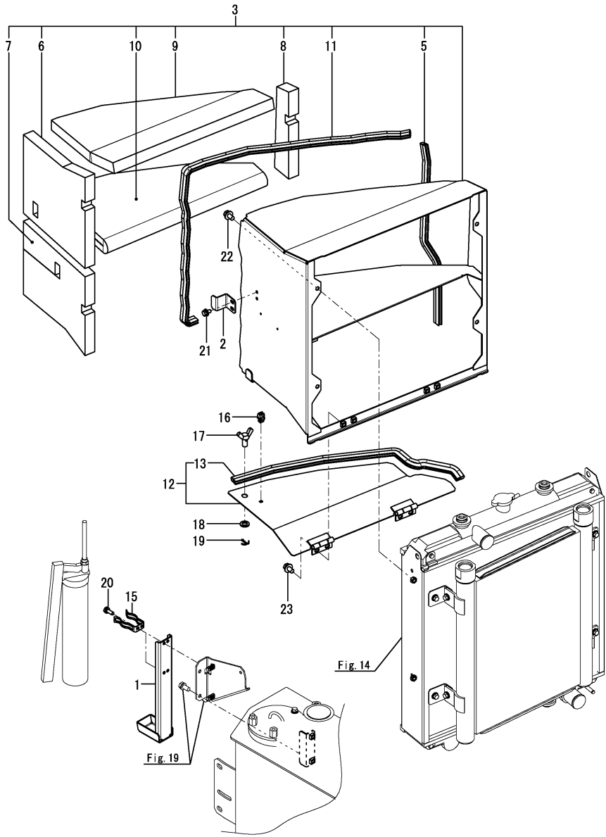
Fig.16. DUCT
