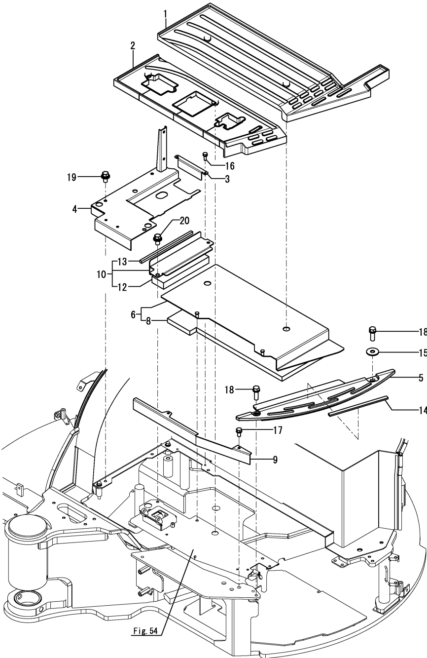
Fig.78. STEP(CABIN)
