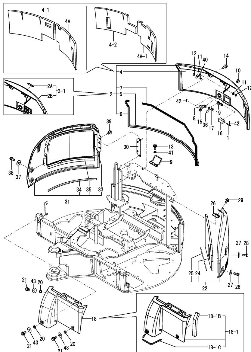
Fig.36. BONNET
