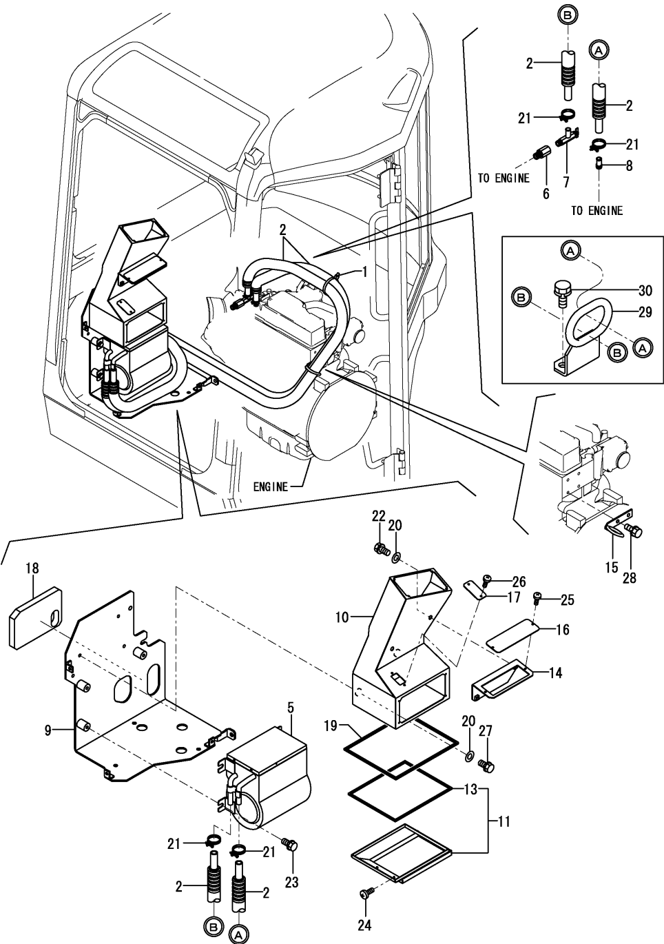
Fig.100. (15A)HEATER(TO M53273)
