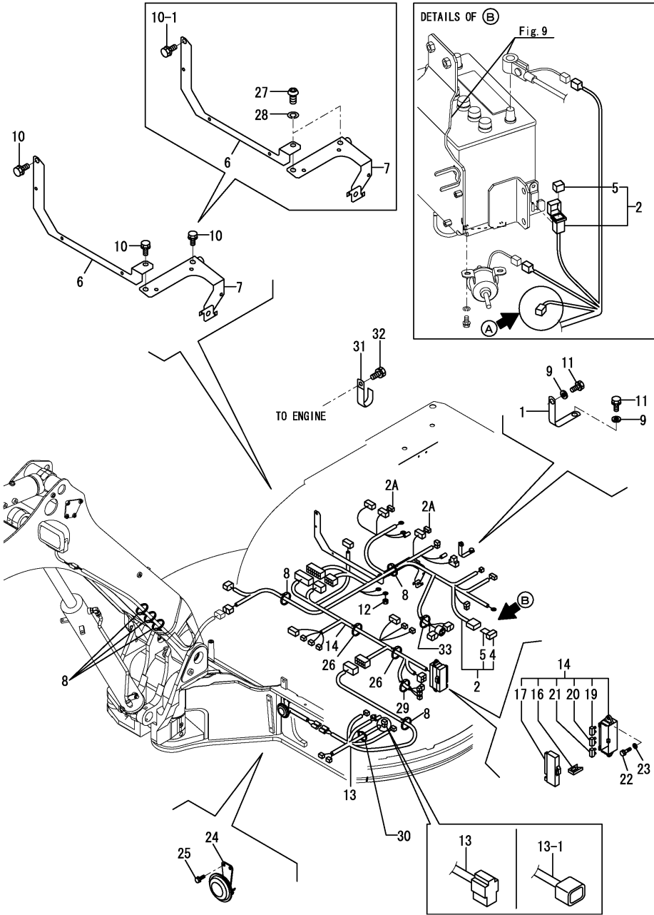
Fig.10. WIRING
