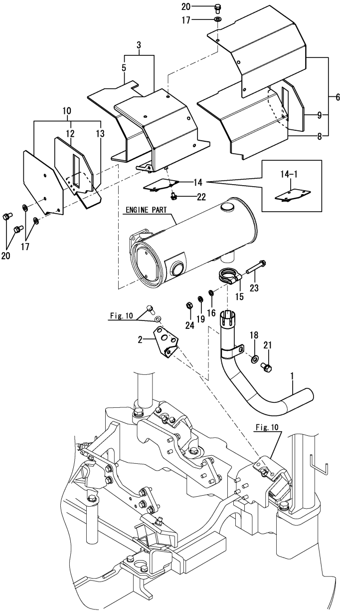
Fig.7. MUFFLER
