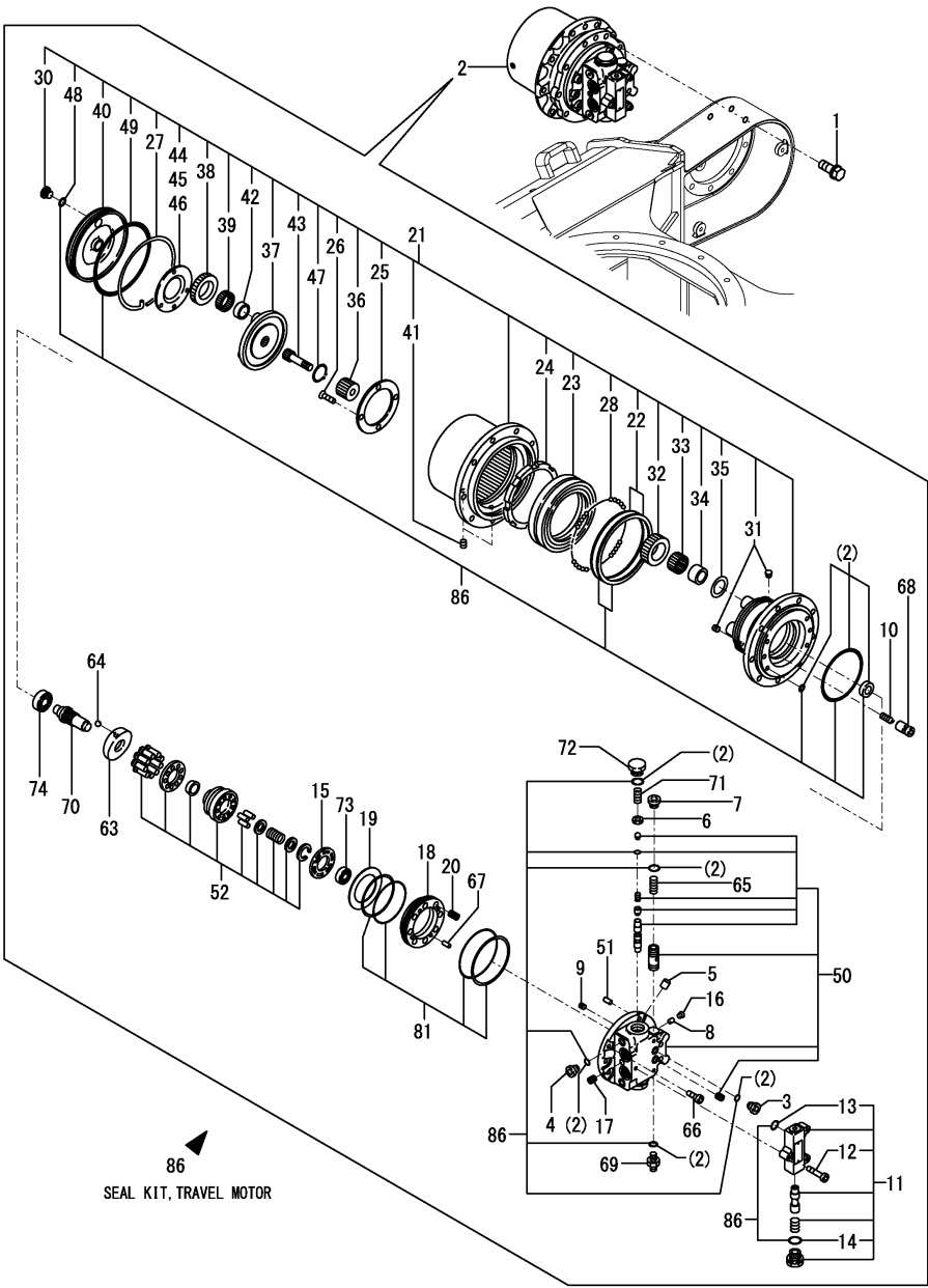
Fig.92. TRAVEL MOTOR
