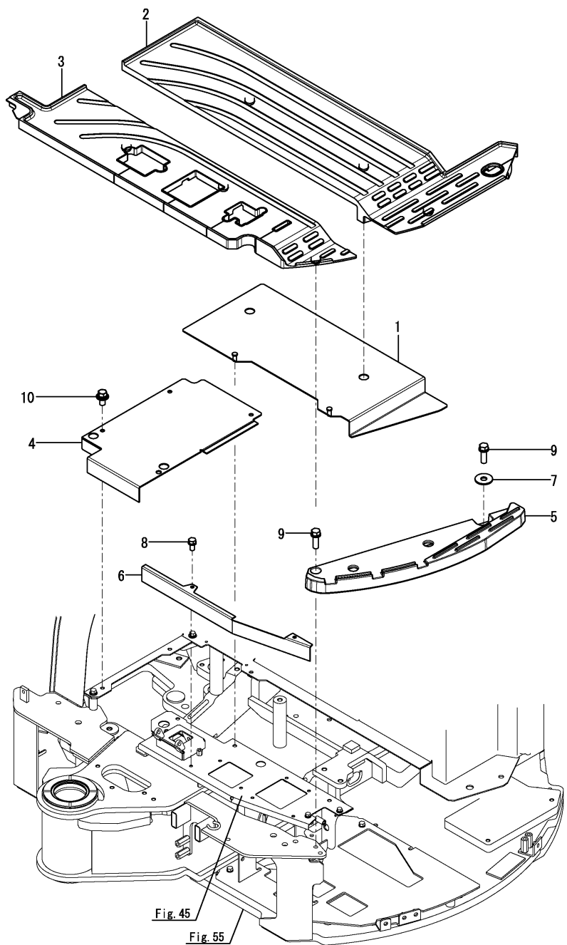
Fig.64. STEP(CANOPY)
