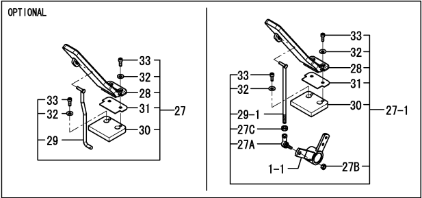
Fig.5. FOOT ACCELERATOR
