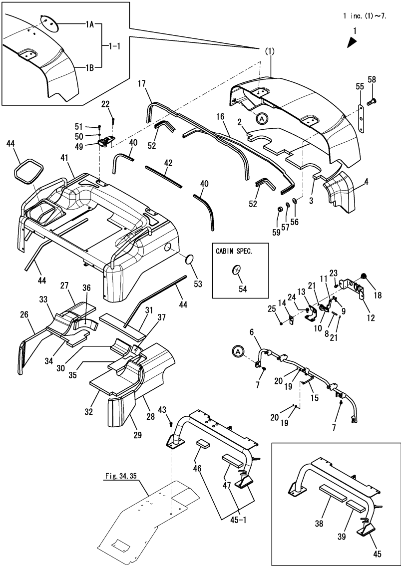
Fig.38. BONNET
