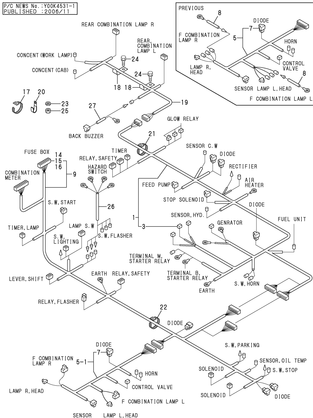
Fig.10. WIRING
