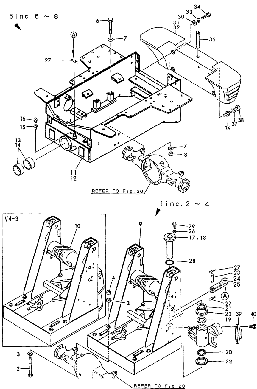
Fig.31 FRAME
