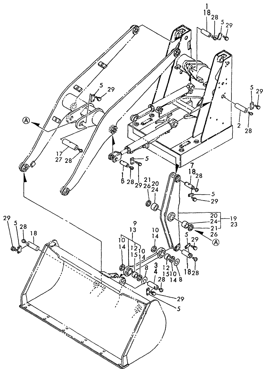
Fig. 48 LOADER LINK
