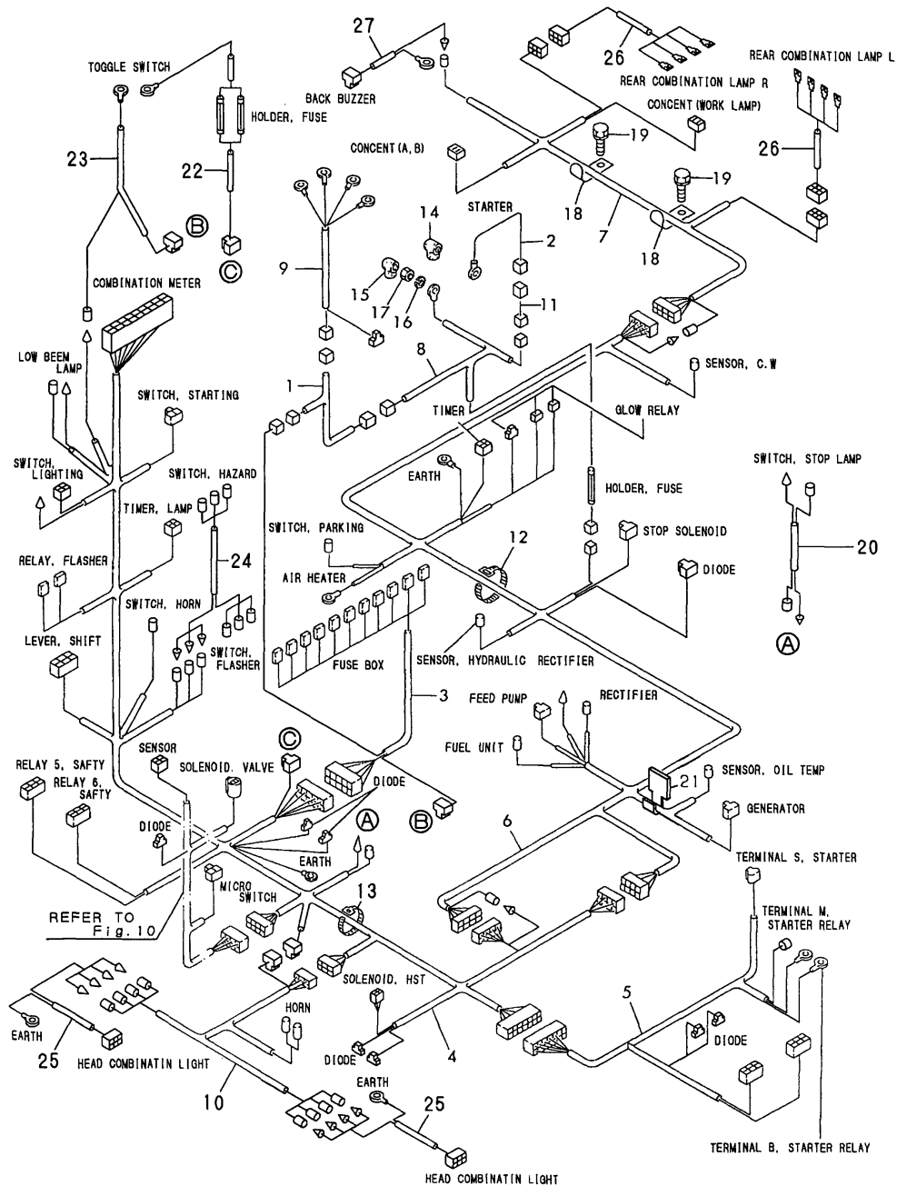
Fig. 11 WIRING
