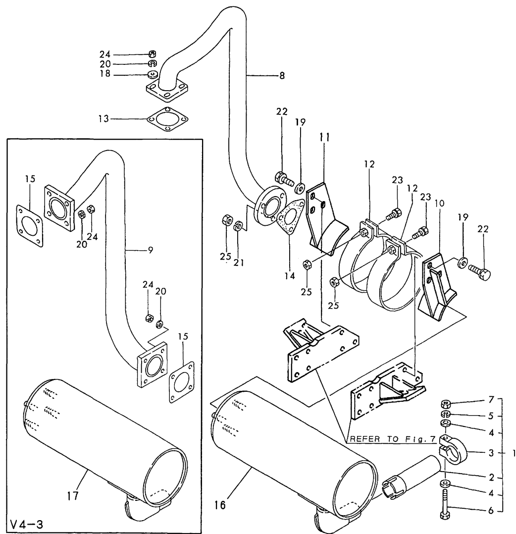
Fig.4 SILENCER
