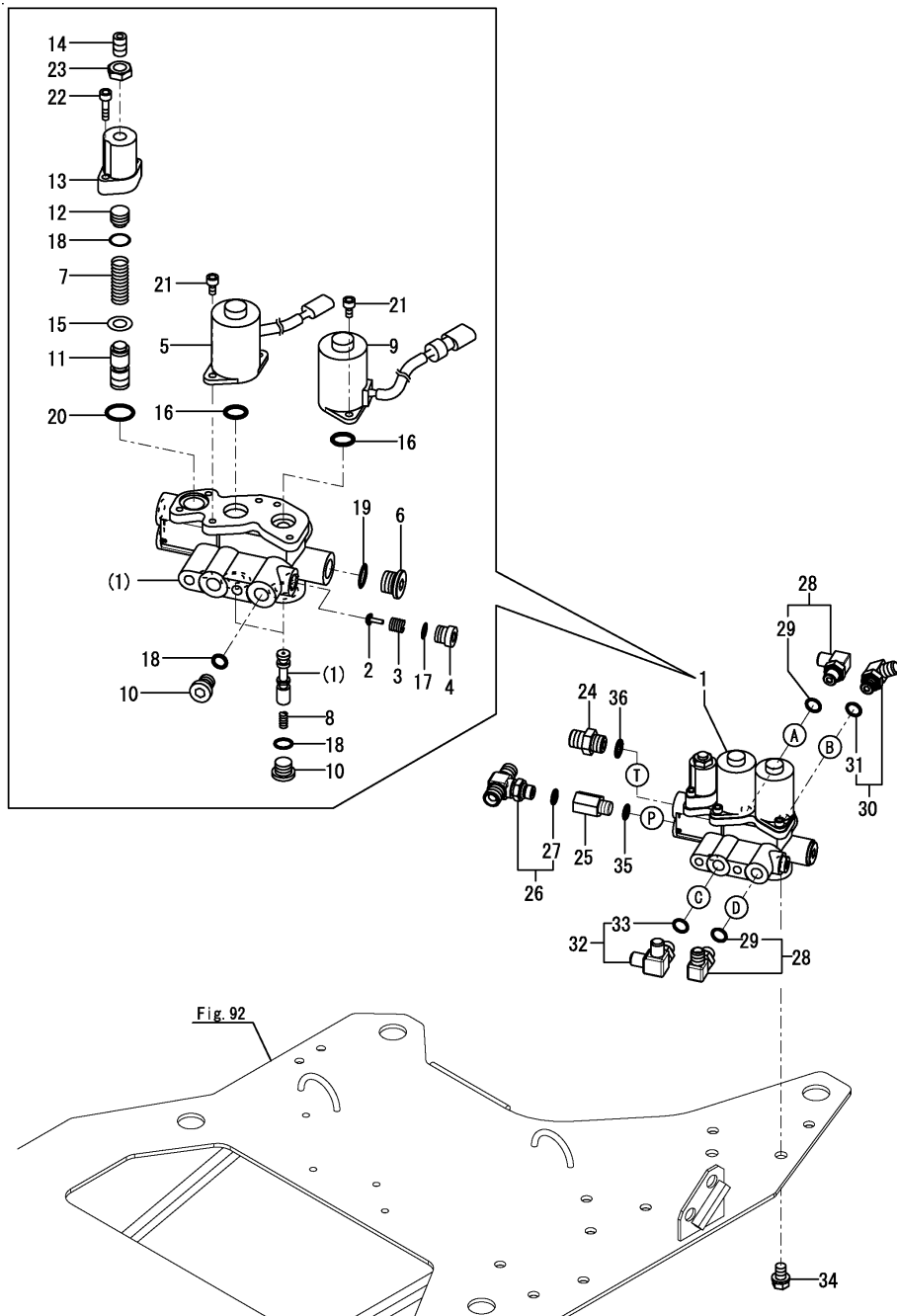
Fig.115. SOLENOID VALVE(PILOT).
