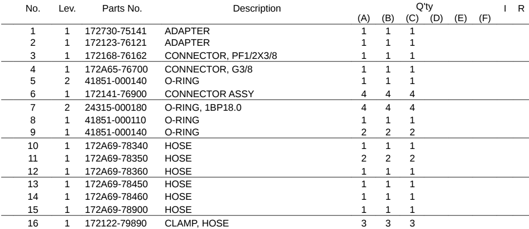
(A)=SV100-2B(US) (B)=SV100-2B(AS) (C)=SV100-2B(NZ)
