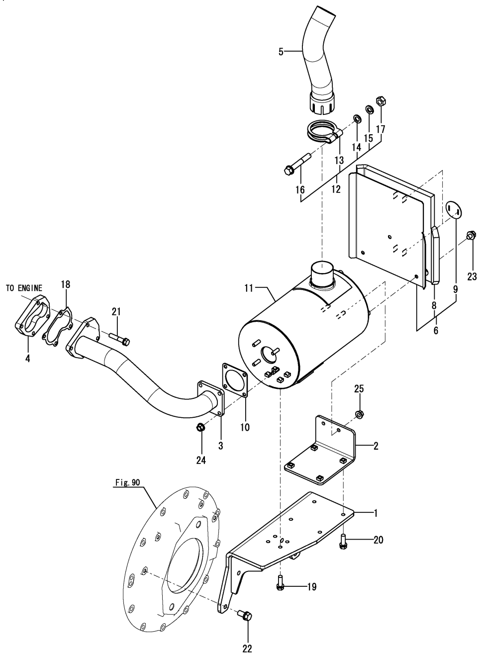
Fig.6. SILENCER
