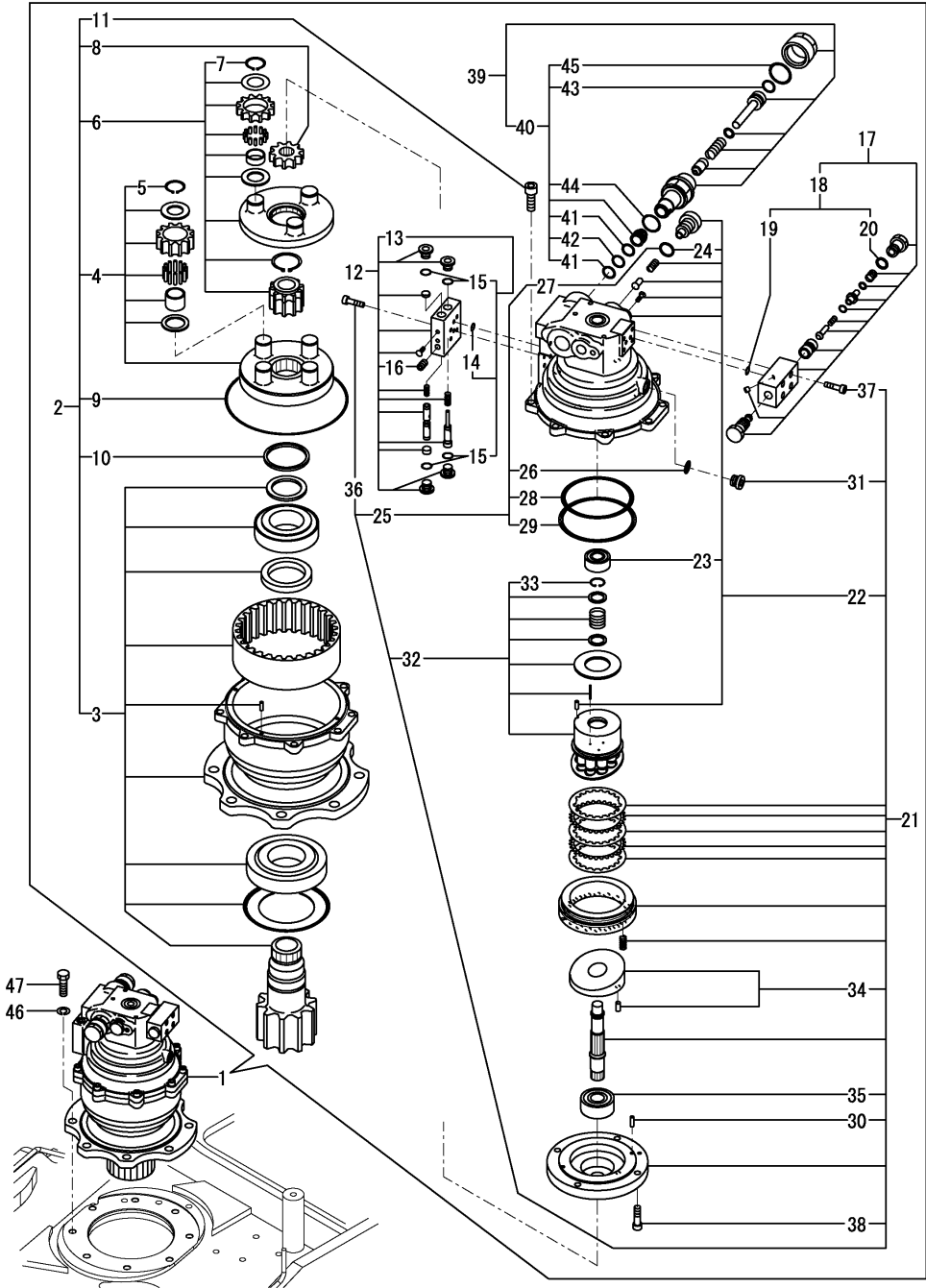
Fig.100. TURNING MOTOR
