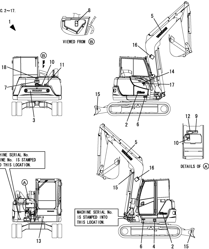
Fig.1. LABEL(EXTERIOR)(TO MBF000)
