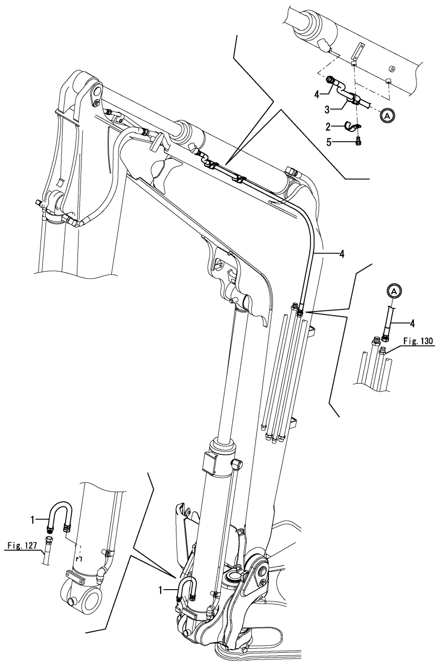
Fig.133. BOOM (3)
