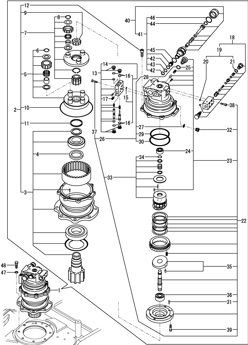
Fig.96. TURNING MOTOR
