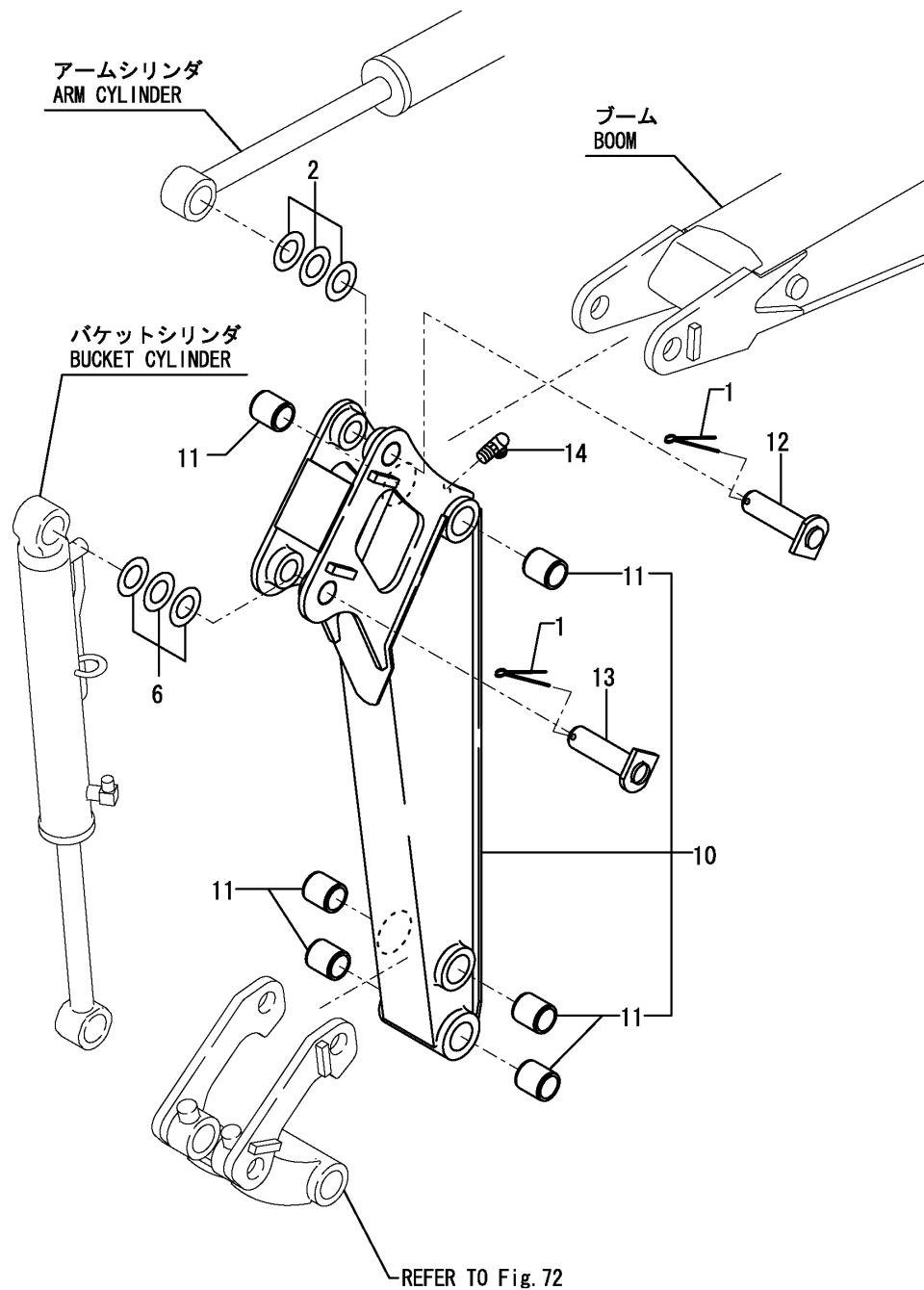
Fig.70. ARM
