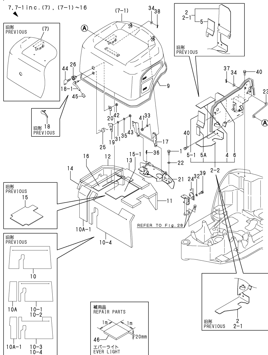
Fig.30. BONNET
