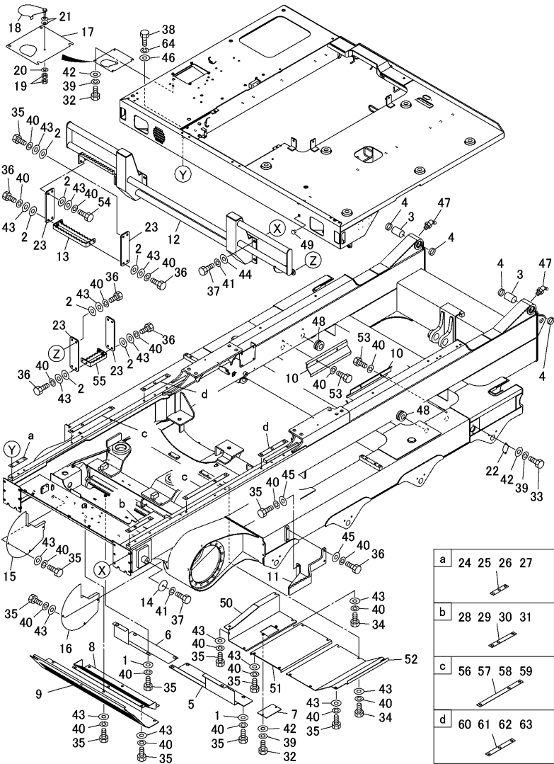
Fig.1. FRAME
