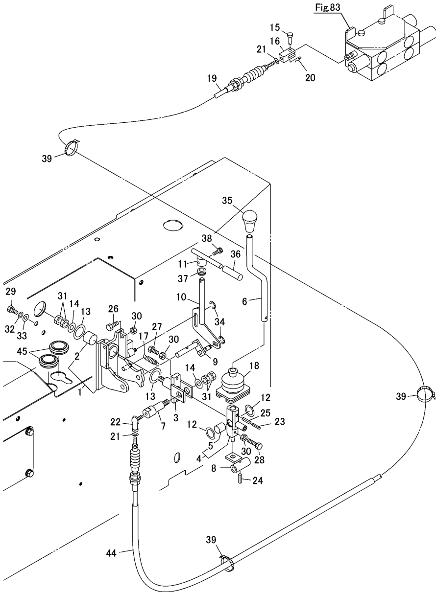
Fig.15. DUMP LEVER
