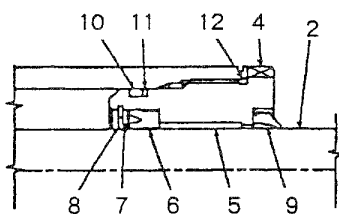
シリンダヘッド部詳細
