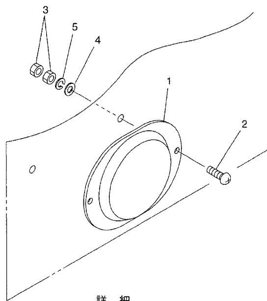
“A” 詳細 DETAIL
