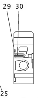
"K" 詳細 DETAIL
