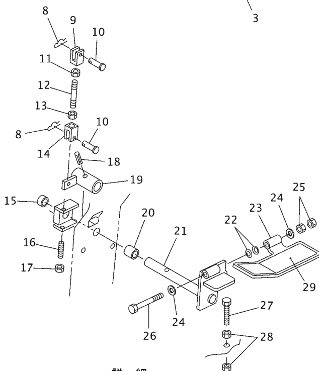
"B" 詳細 DETAIL
