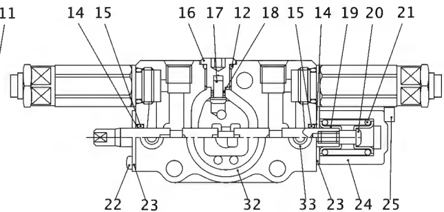
"B" 詳細 DETAIL
