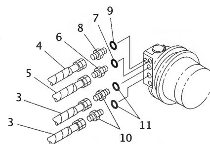
"B" 詳細 DETAIL
