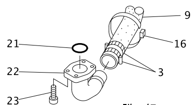
"B" 詳細 DETAIL
