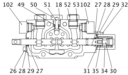
"F-F" 断面 SECTION
