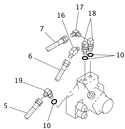
"B" 詳細 DETAIL
