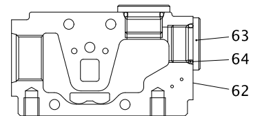
"K-K" 断面 SECTION
