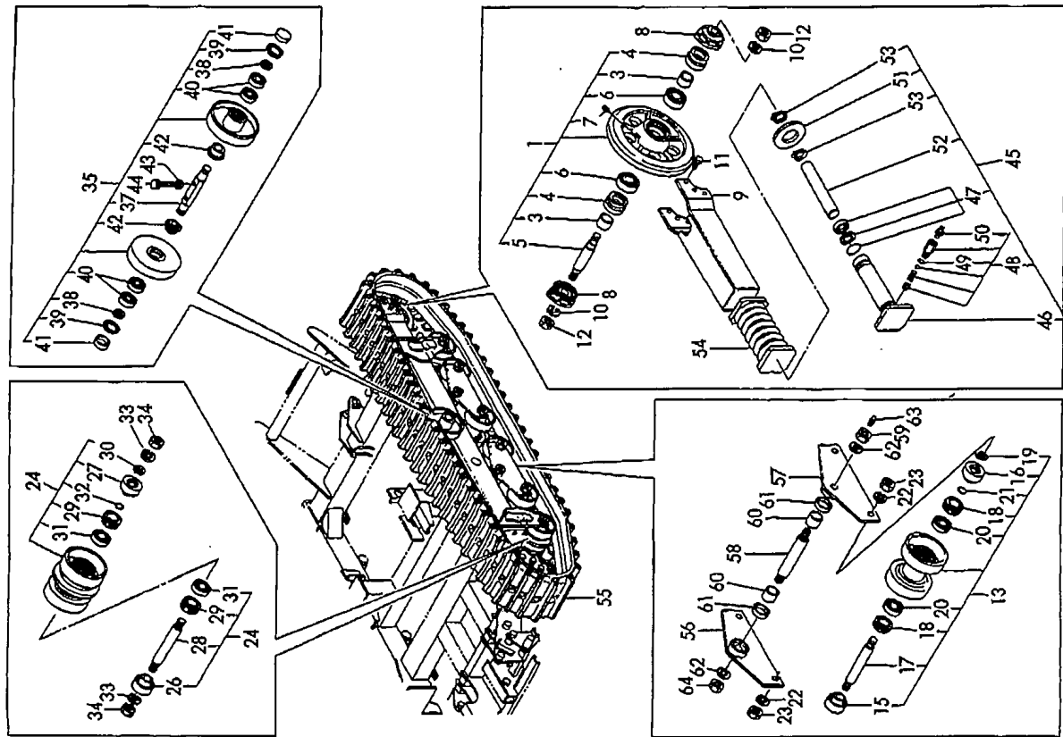
Fig.45 ローフ&アジャスト ROLLER & ADJUST
