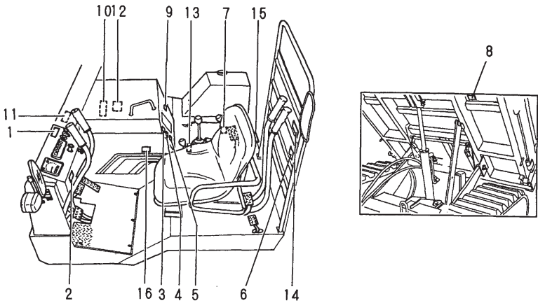
Fig.86 安全銘板 (C30R) SAFETY LABEL (C30R)
