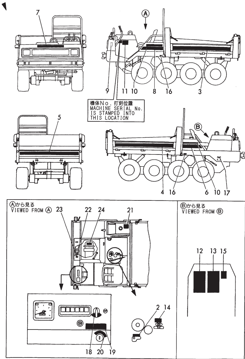
Fig.5 銘板 (C25W) (UK) LABEL (C25W) (UK)
