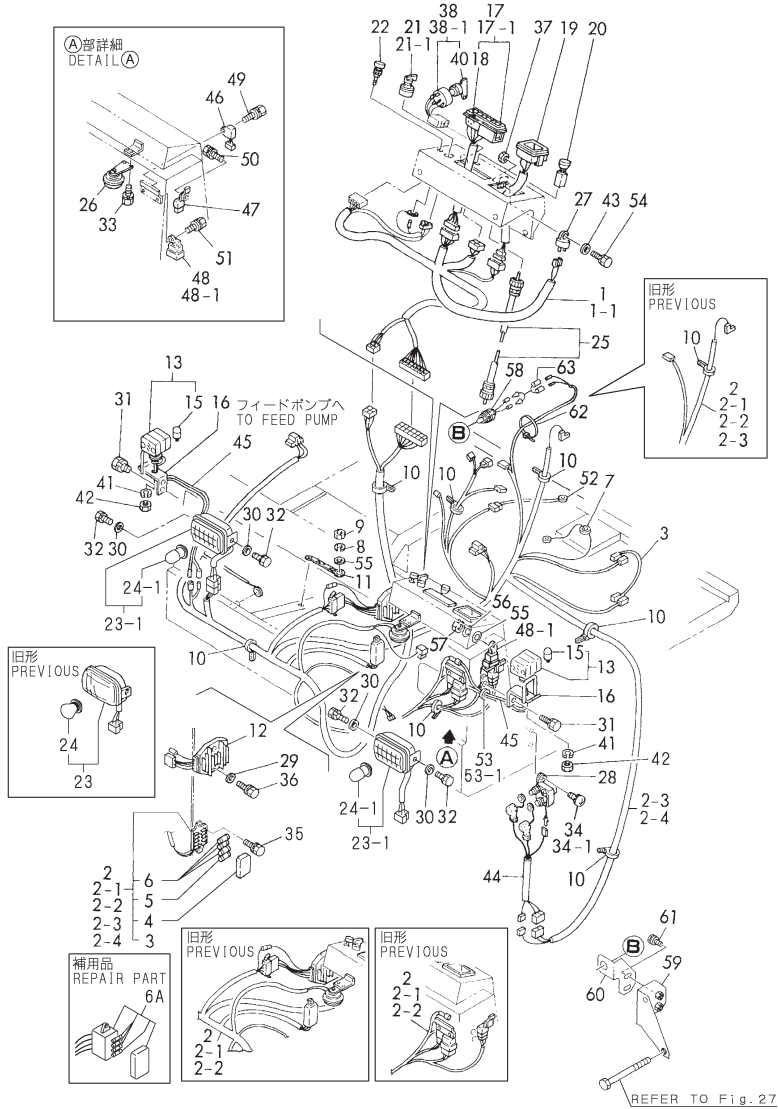
Fig.25 電装品 ELECTRIC PART
