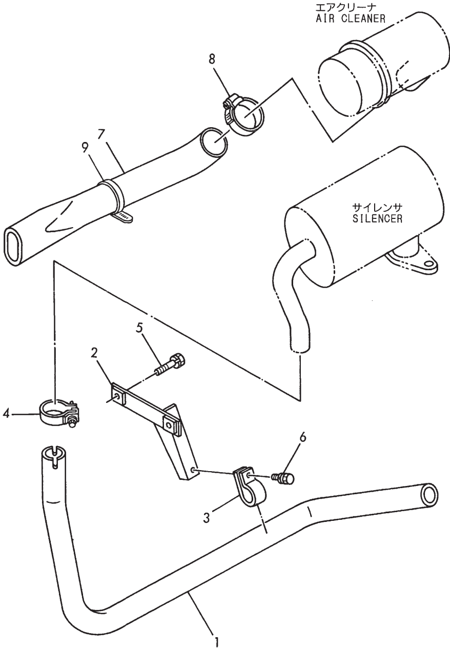
Fig. 14 吸気管&排気管 (C20R) SUC. PIPE & EXH. PIPE (C20R)
