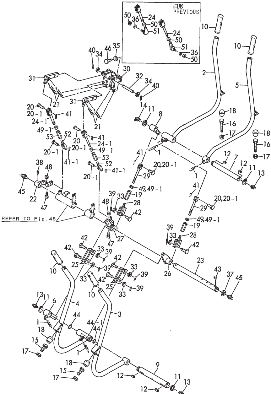
Fig.52 ステアリングレバー (C20R) STEERING LEVER (C20R)
