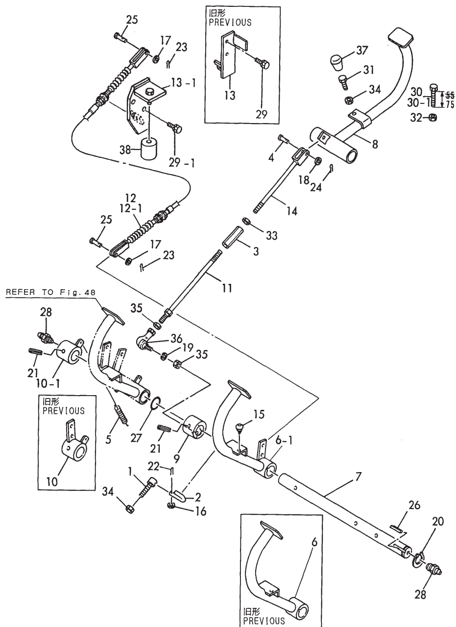
Fig. 46 操縦装置 (クラッチペダル) (C20R) CONTROL EQUIPMENT (CLUTCH PEDAL) (C20R)
