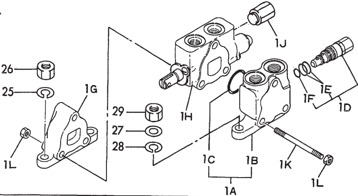
Fig.74 コントロールバルブ (C20R) CONTROL VALVE (C20R)
