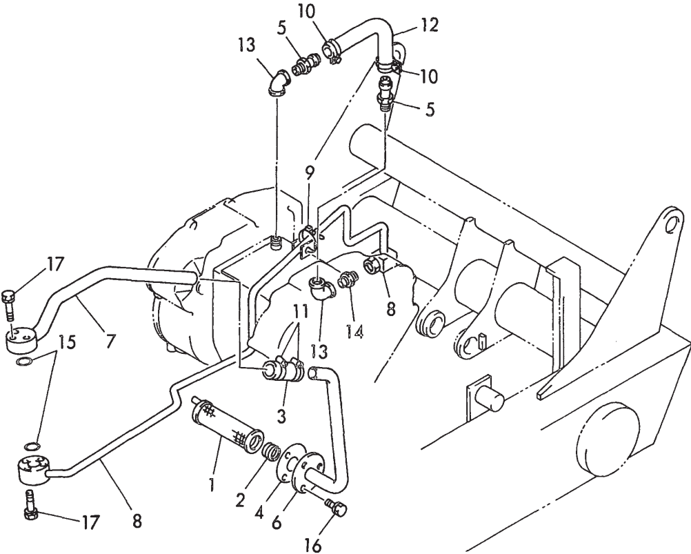
Fig.68 油圧配管 (C30R-F) HYD.OIL PIPING (C30R-F)
