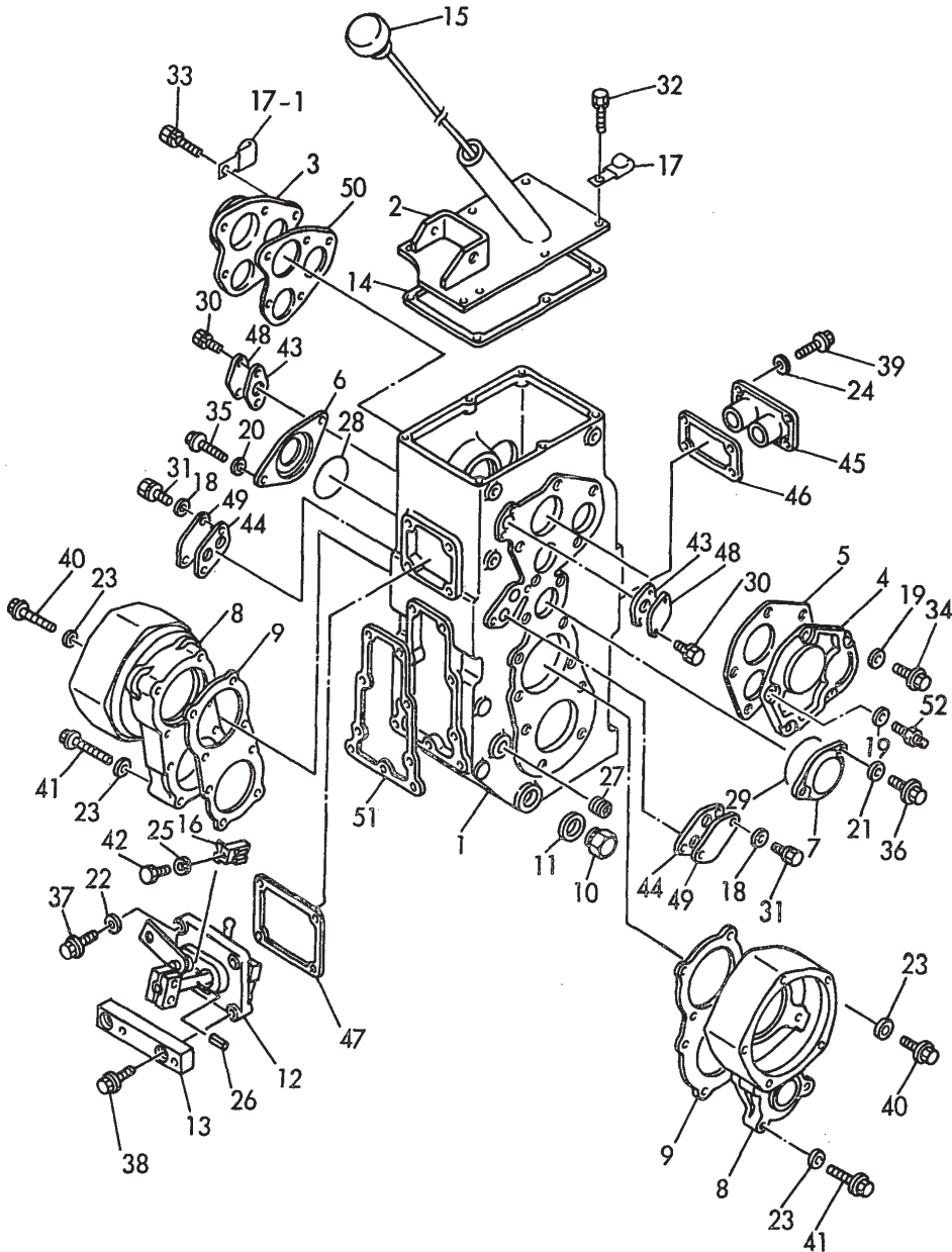
Fig.28 トランスミッションケース (C20R) TRANSMISSION CASE (C20R)
