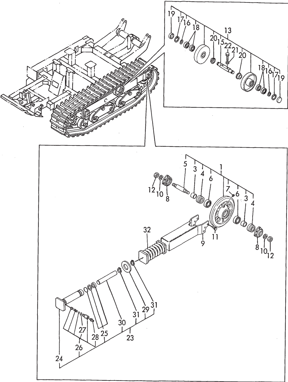
Fig.43 キャリヤローラ&アジャスト (C20R) CARRIER ROLLER & ADJUST (C20R)
