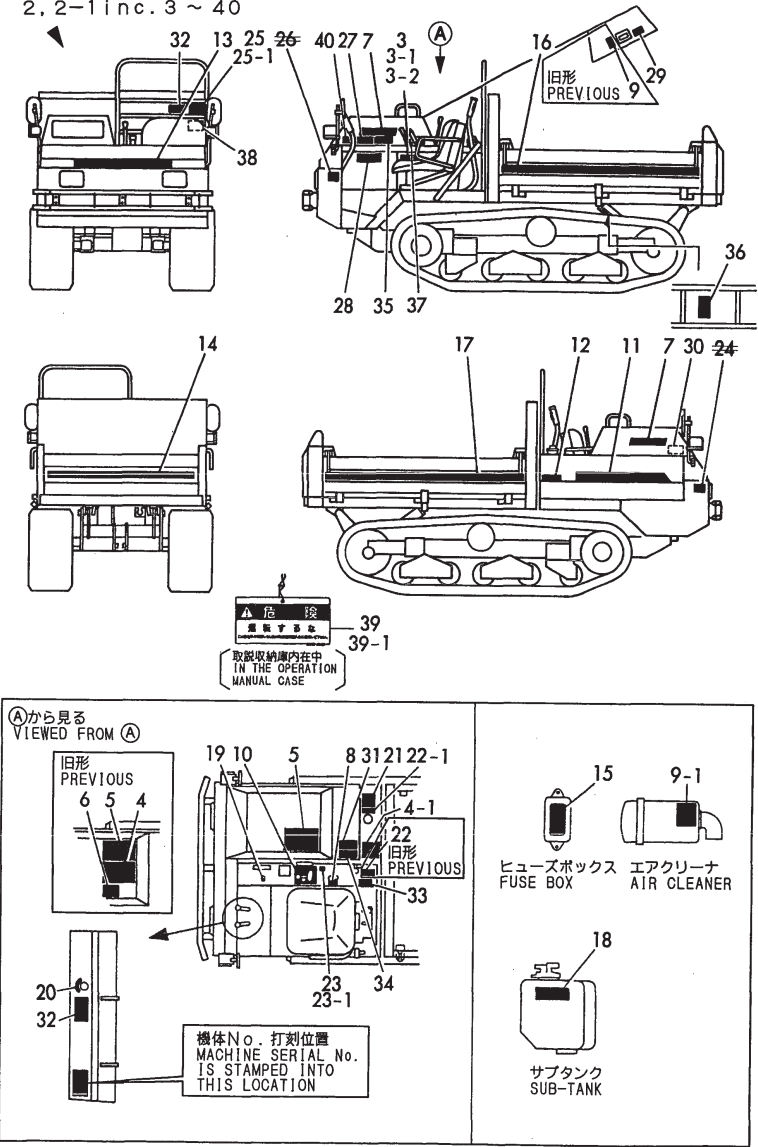
Fig.1 銘板 (C20R) (JP) LABEL (C20R) (JP)
