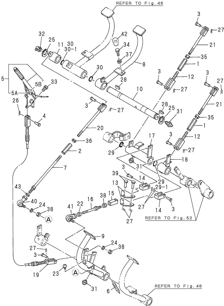
Fig.48 操縦装置 (ブレーキペダル) (C20R) CONTROL EQUIPMENT (BRAKE PEDAL) (C20R)
