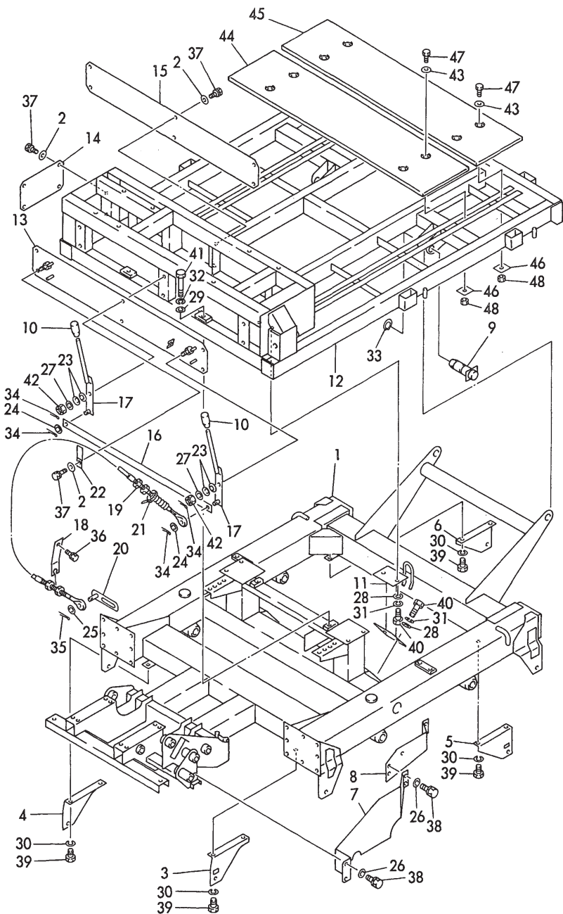
Fig.58 リヤフレーム (C30R-1K) REAR FRAME (C30R-1K)
