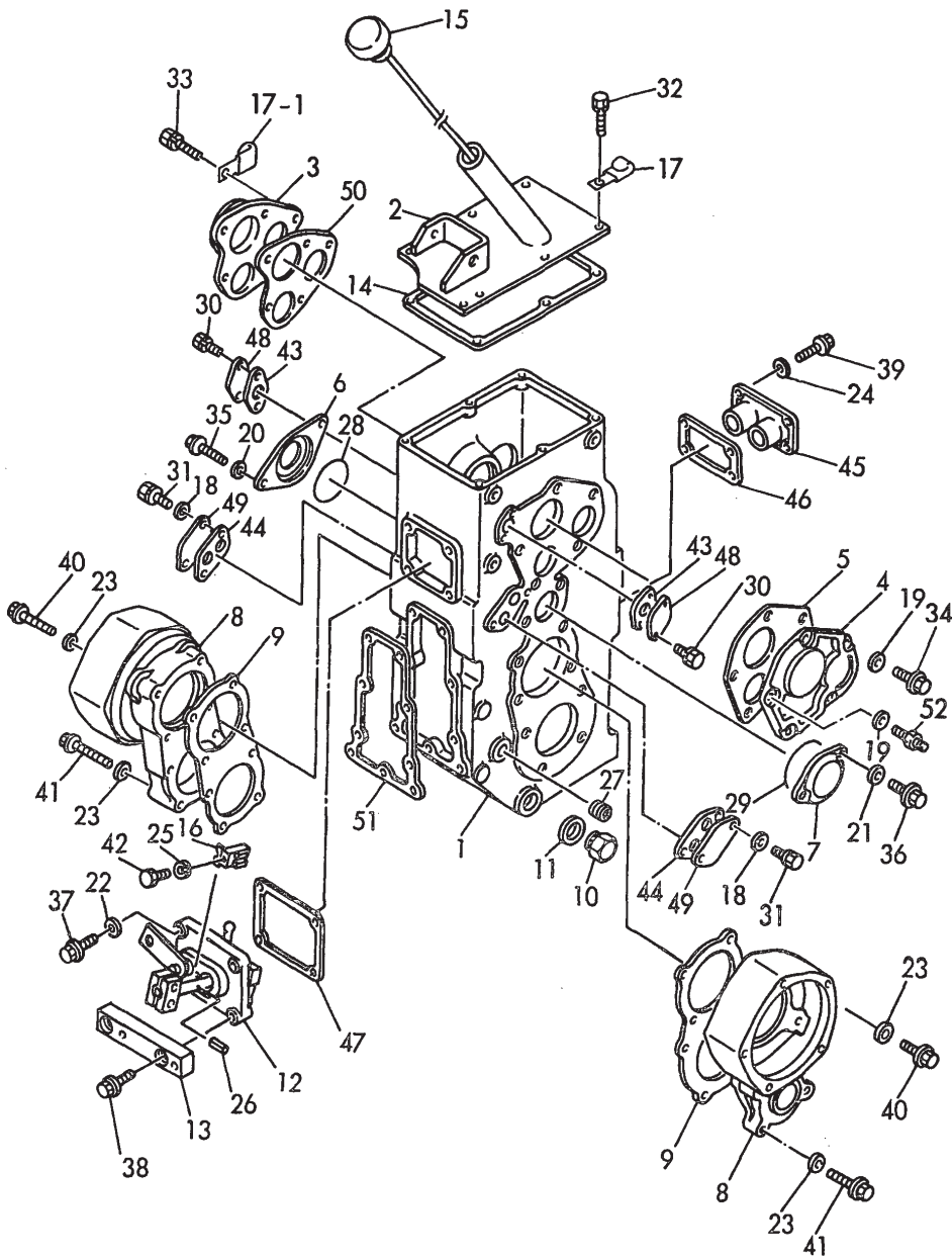
Fig.28 トランスミッションケース (C20R) TRANSMISSION CASE (C20R)
