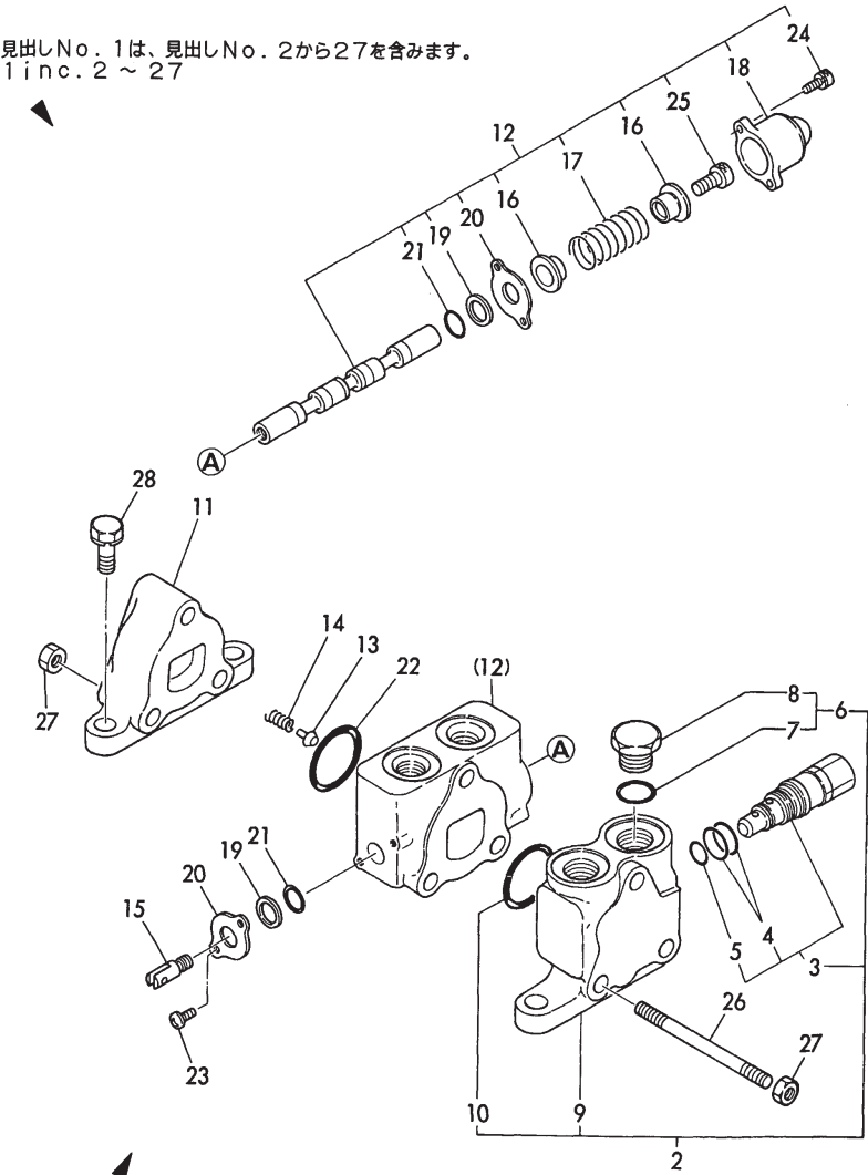
Fig.76 コントロールバルブ (C25W) (C30R) CONTROL VALVE (C25W) (C30R)
