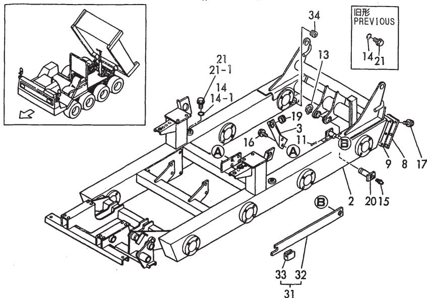
Fig.57 リヤフレーム (C25W) (C30R) REAR FRAME (C25W) (C30R)
