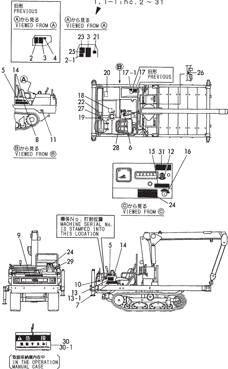
Fig. 12 銘板 (C30R-2K) LABEL (C30R-2K)
