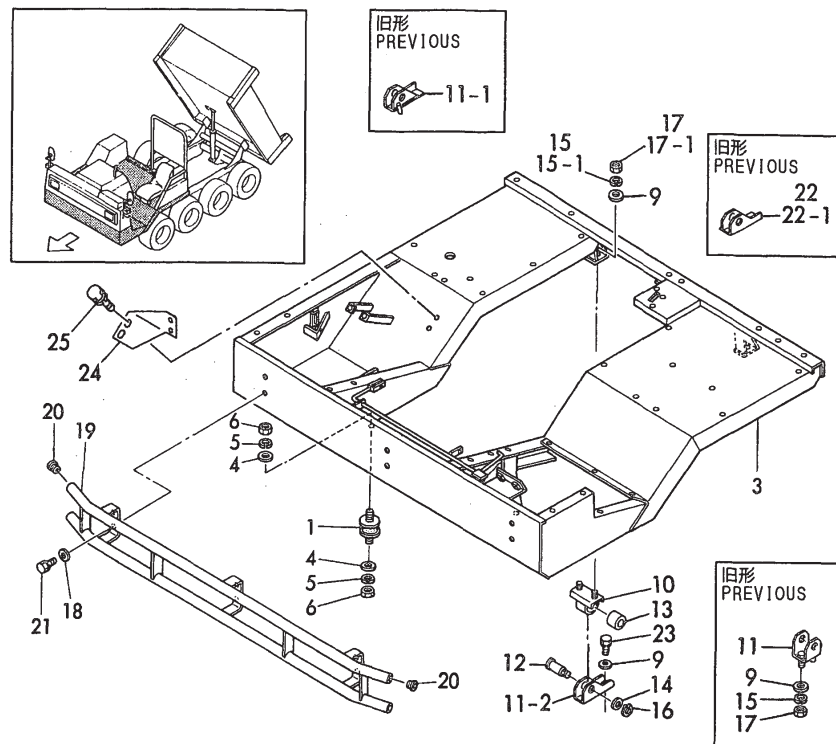
Fig.61 フロントフレーム FRONT FRAME
