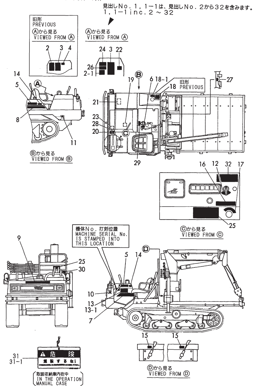
Fig. 11 銘板 (C30R-1K) LABEL (C30R-1K)
