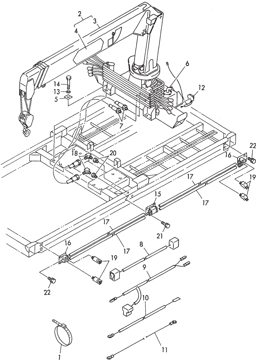
Fig.84 クレーン (C30R-2K) CRANE (C30R-2K)
