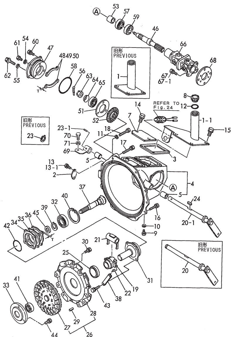
Fig. 26 メインクラッチ (C20R) MAIN CLUTCH (C20R)
