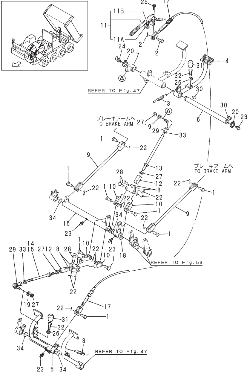
Fig.49 操縦装置 (ブレーキペダル) CONTROL EQUIPMENT (BRAKE PEDAL)
