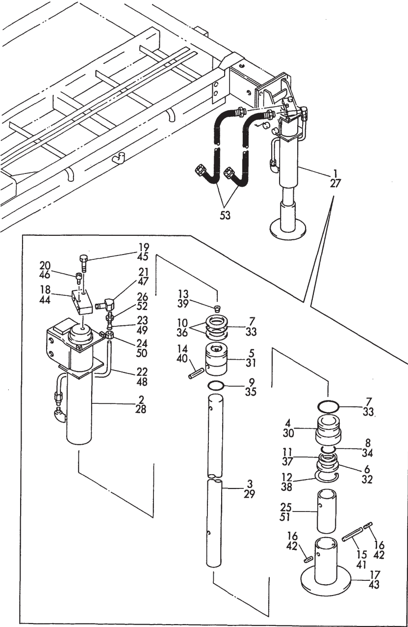
Fig.82 アウトリガリヤ (C30R-2K) OUTRIGGER REAR (C30R-2K)
