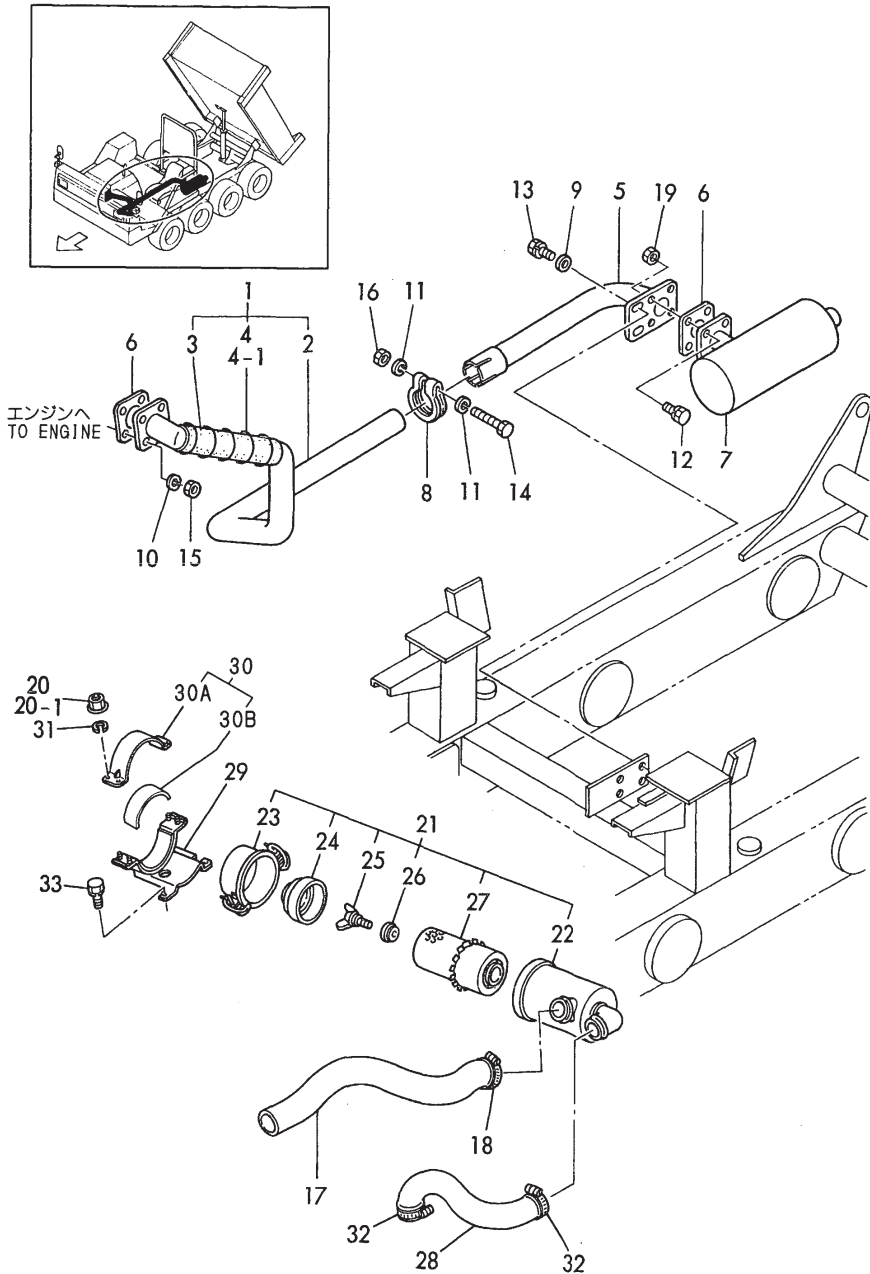
Fig. 15 エアクリーナ&サイレンサ AIR CLEANER & SILENCER
