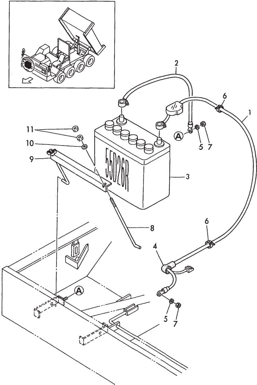
Fig.23 バッテリ BATTERY
