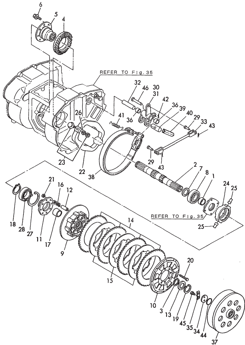
Fig.38 クラッチ&ブレーキ (C30R) CLUTCH & BRAKE (C30R)
