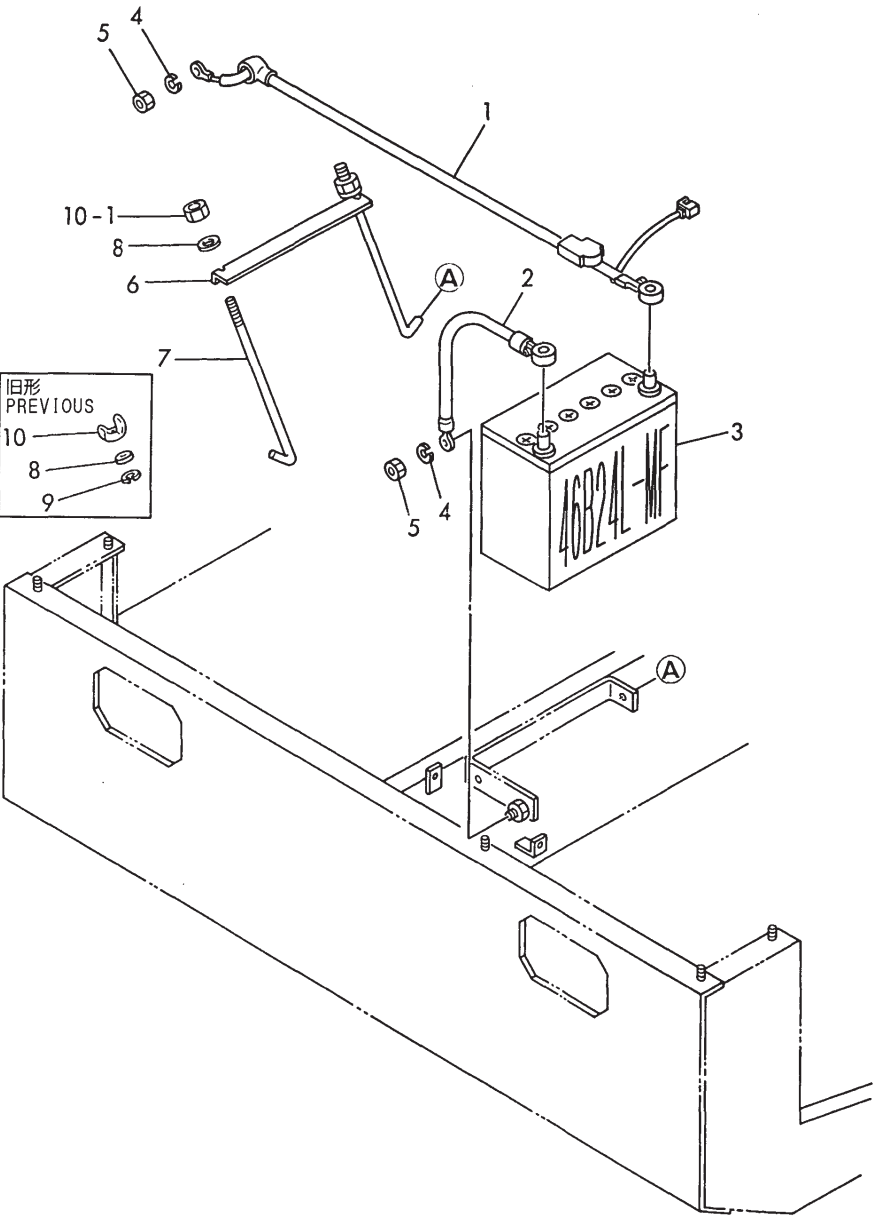
Fig.22 バッテリ (C20R) BATTERY (C20R)
