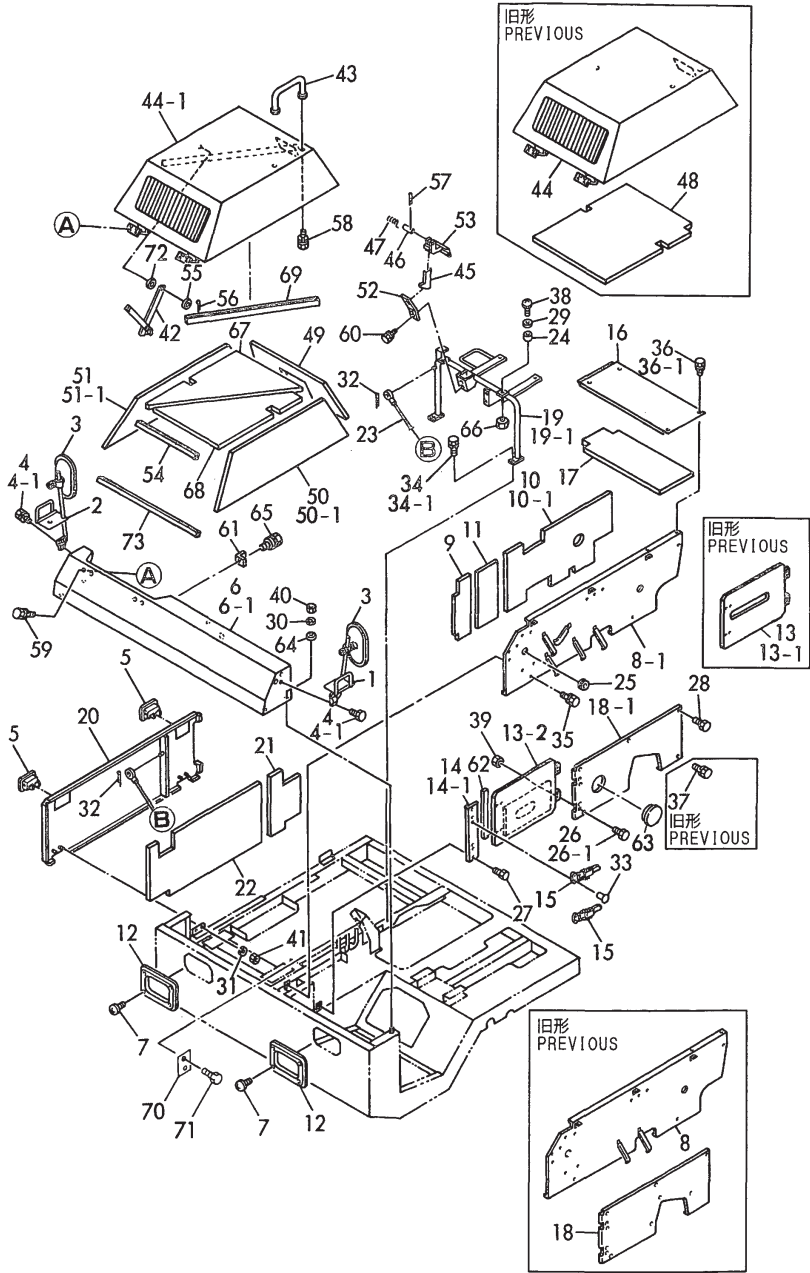
Fig.62 ボンネット (C20R) BONNET (C20R)
