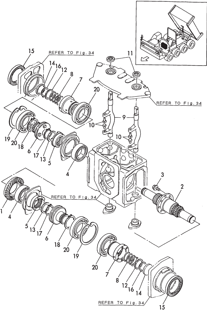
Fig.37 クラッチ&ブレーキ (C25W) CLUTCH & BRAKE (C25W)
