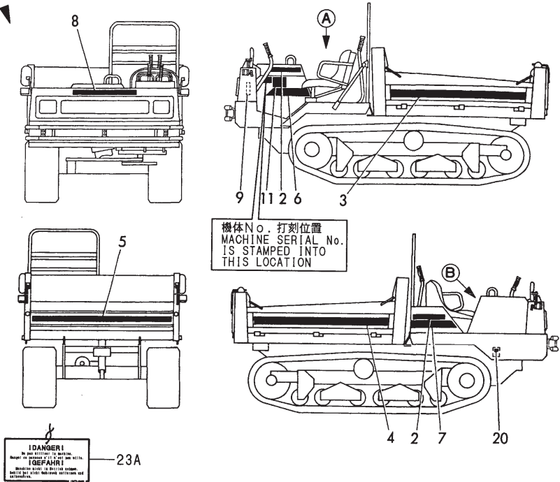
Fig.9 銘板 (C30R) (FA) LABEL (C30R) (FA)
