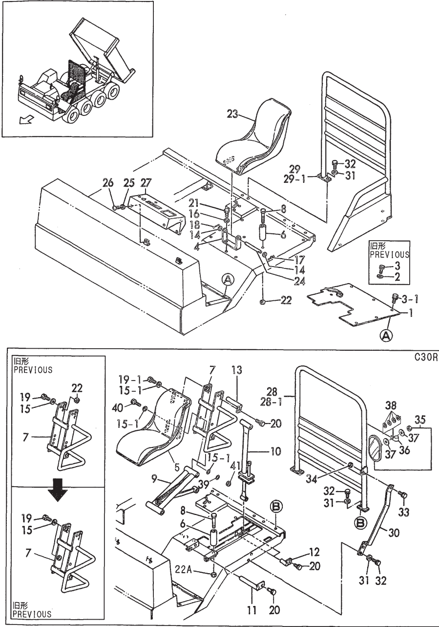
Fig.65 シート&ステップ SEAT & STEP
