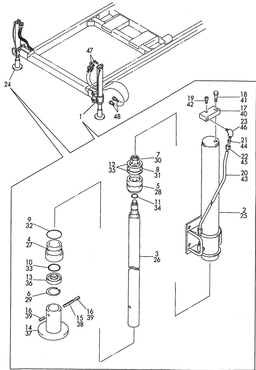
Fig.81 アウトリガフロント (C30R-2K) OUTRIGGER FRONT (C30R-2K)
