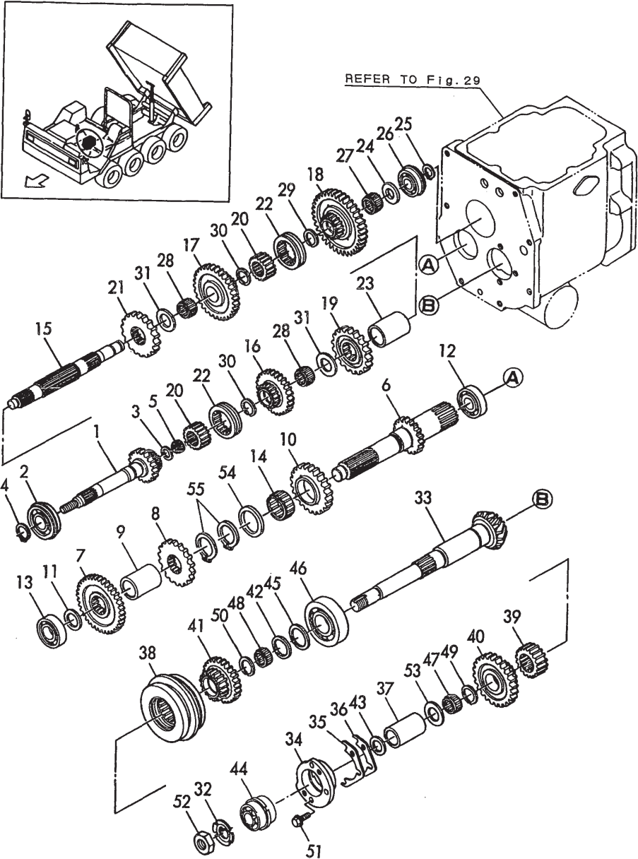
Fig.31 トランスミッションギヤ TRANSMISSION GEAR
