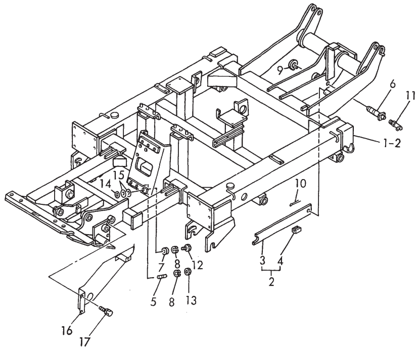
Fig.56 リヤフレーム (C20R) REAR FRAME (C20R)
