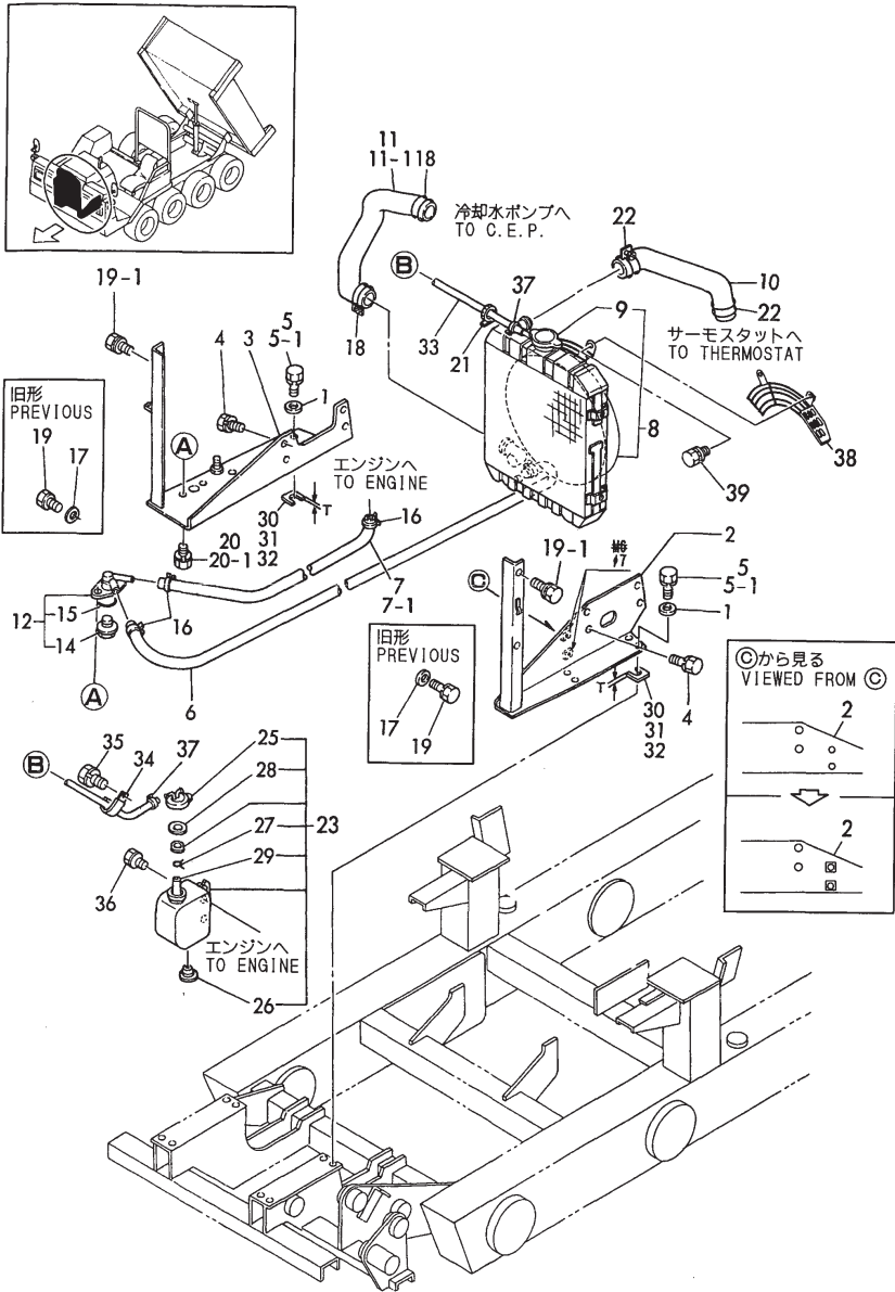
Fig. 19 エンジンマウント&ラジエータ ENGINE MOUNT & RADIATOR
