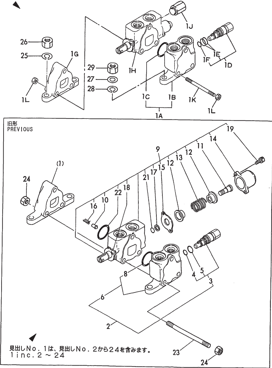
Fig.74 コントロールバルブ (C20R) CONTROL VALVE (C20R)
