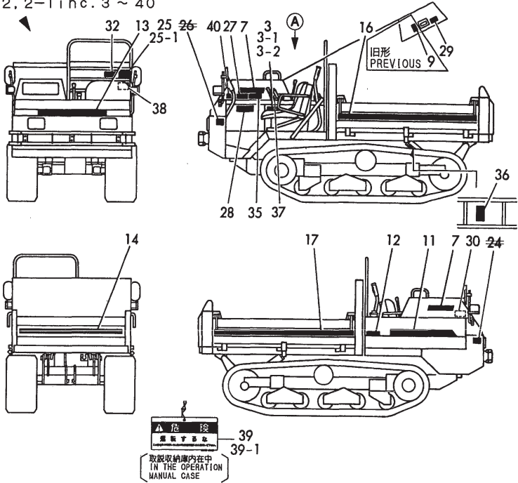
Fig.1 銘板 (C20R) (JP) LABEL (C20R) (JP)
