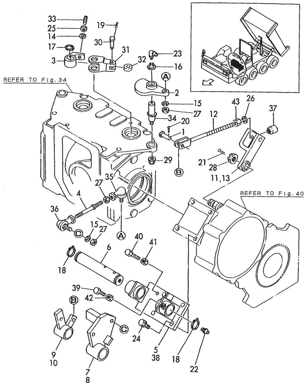
Fig.54 カムレバー (C25W) CAM LEVER (C25W)
