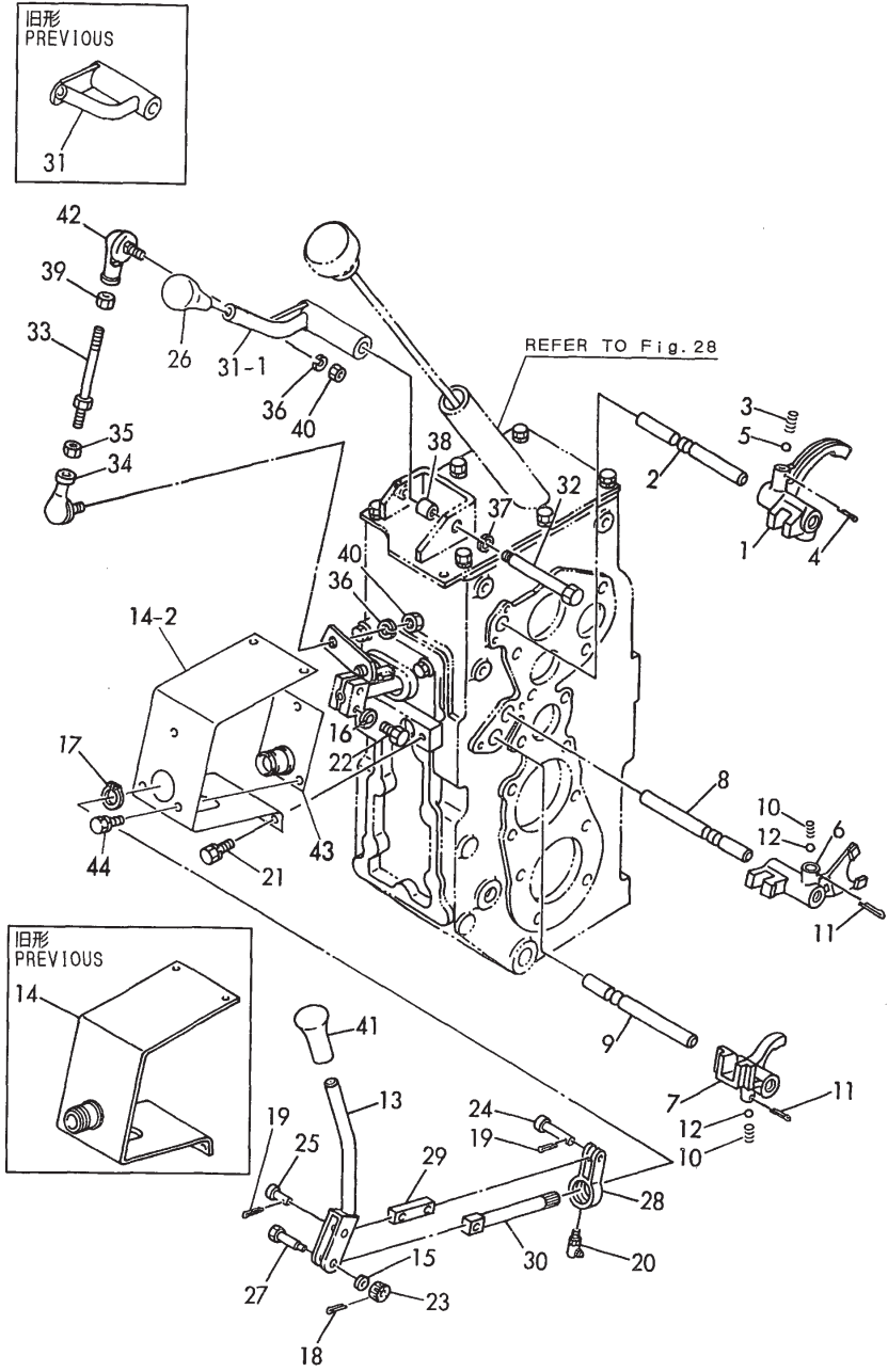
Fig.32 変速レバー (C20R) SPEED CHANGE LEVER (C20R)
