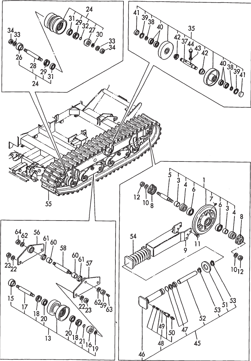
Fig.45 ローラ&アジャスト ROLLER & ADJUST
