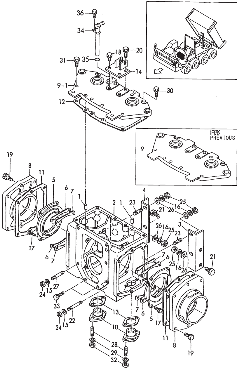
Fig.34 ステアリングケース (C25W) STEERING CASE (C25W)
