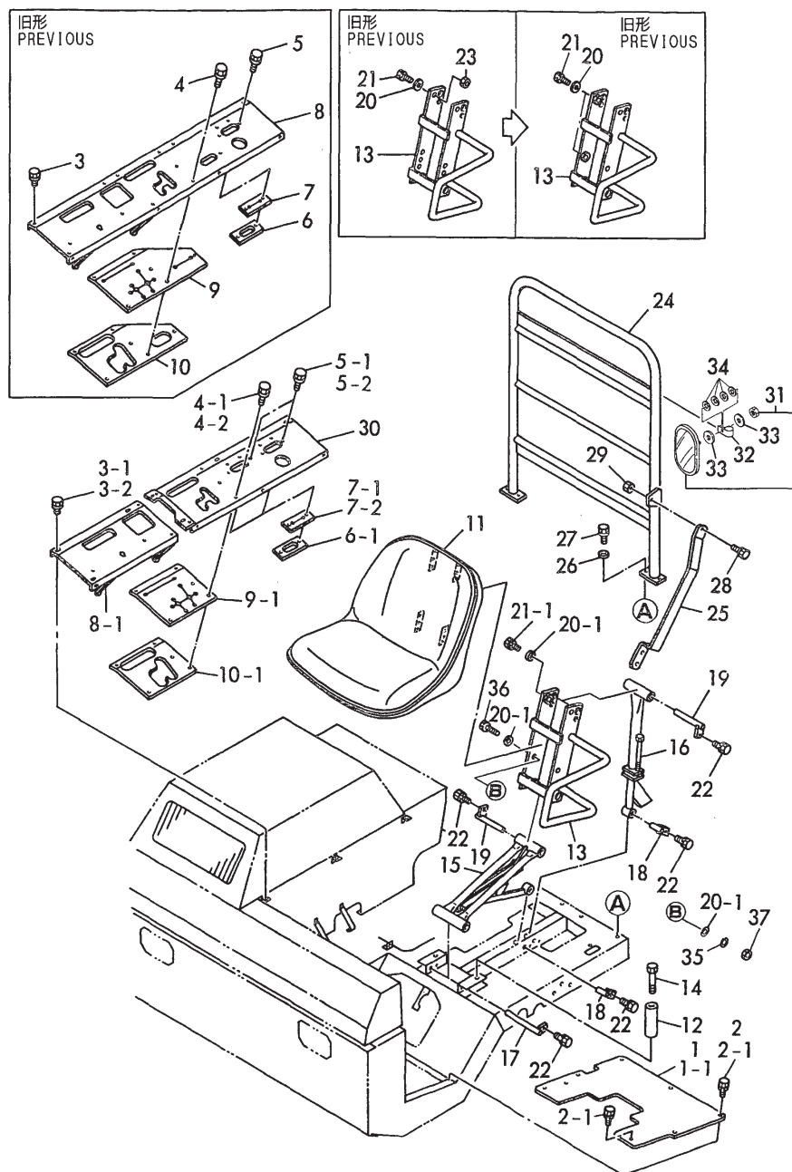
Fig. 64 シート&ステップ (C20R) SEAT & STEP (C20R)
