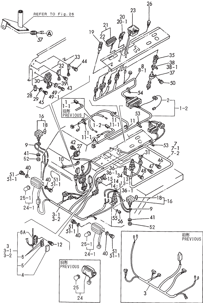
Fig.24 電装品 (C20R) ELECTRIC PART (C20R)
