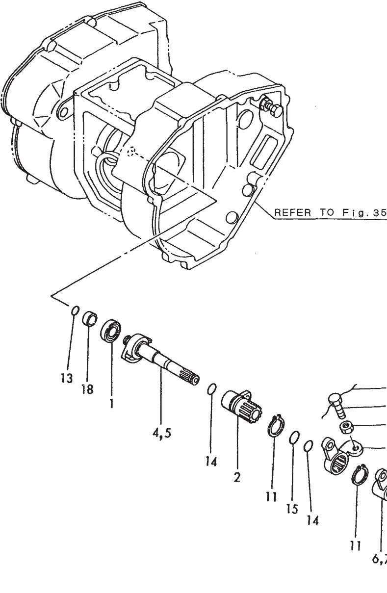
Fig.55 カムレバー (C30R) CAM LEVER (C30R)
