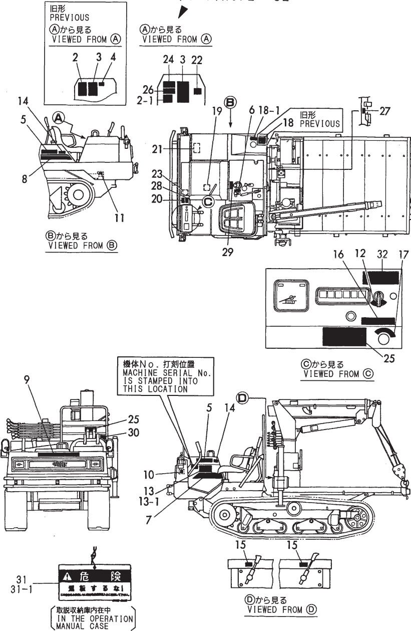
Fig. 11 銘板 (C30R-1K) LABEL (C30R-1K)
