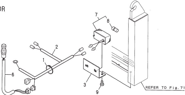
Fig.87 テールランプ (オプション) TAIL LAMP (OPTIONAL)
