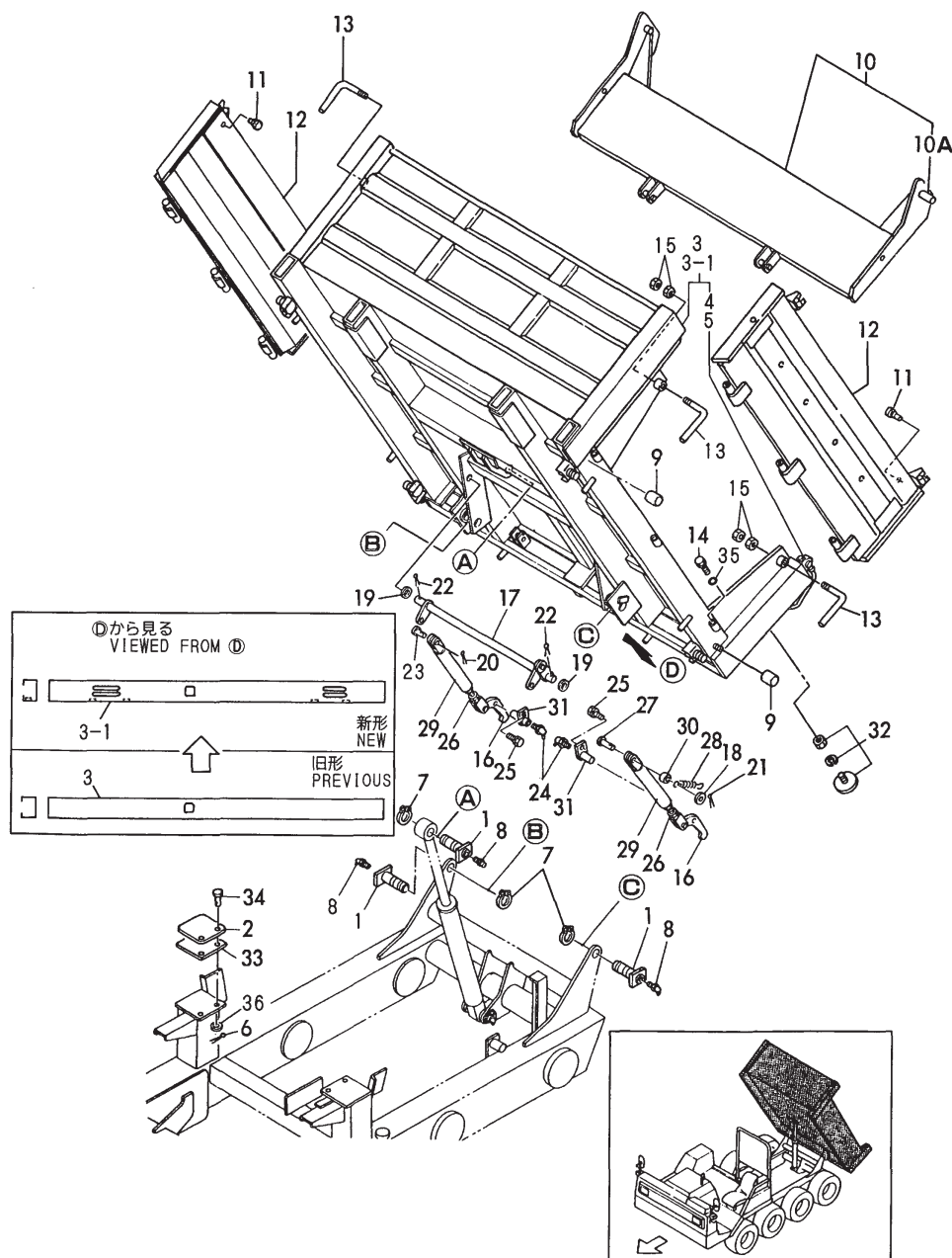
Fig. 72 荷台 (C25W) (C30R) WAGON (C25W) (C30R)
