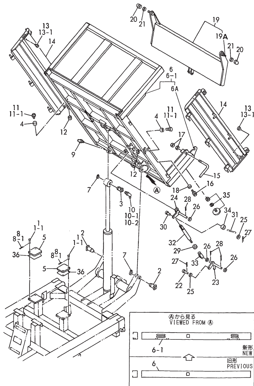
Fig. 71 荷台 (C20R) WAGON (C20R)
