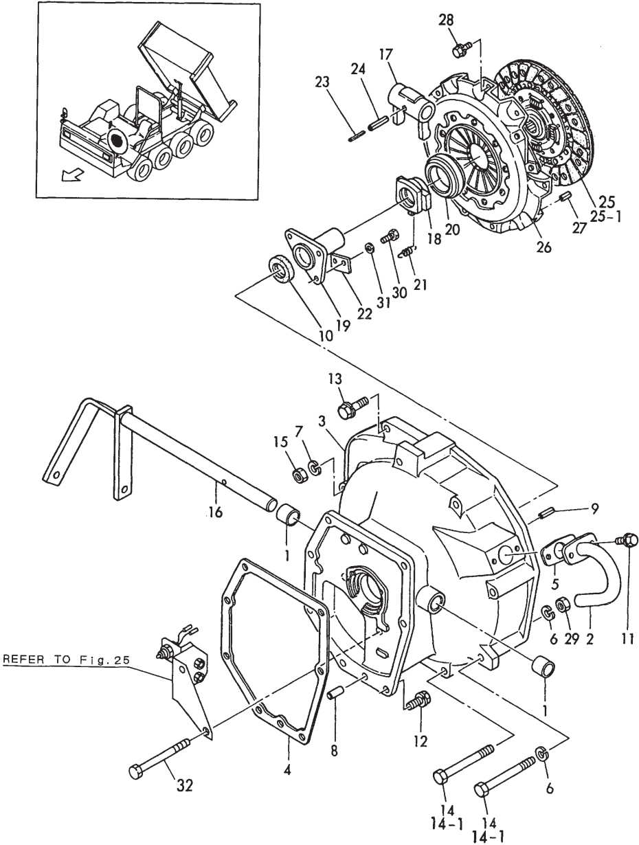
Fig.27 メインクラッチ MAIN CLUTCH
