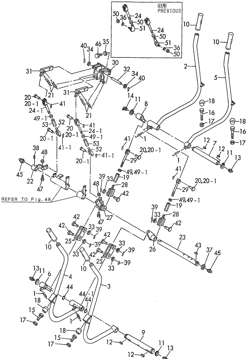
Fig.52 ステアリングレバー (C20R) STEERING LEVER (C20R)
