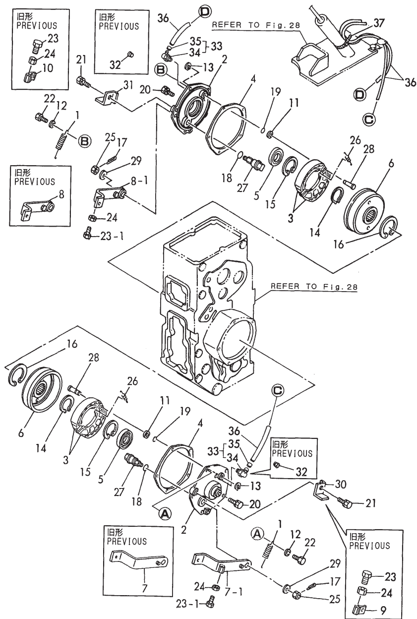
Fig.36 ブレーキ (C20R) BRAKE (C20R)
