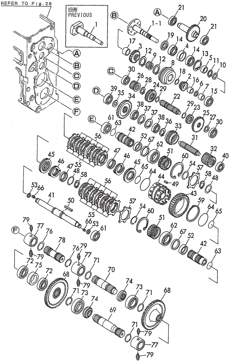
Fig.30 トランスミッションギヤ (C20R) TRANSMISSION GEAR (C20R)
