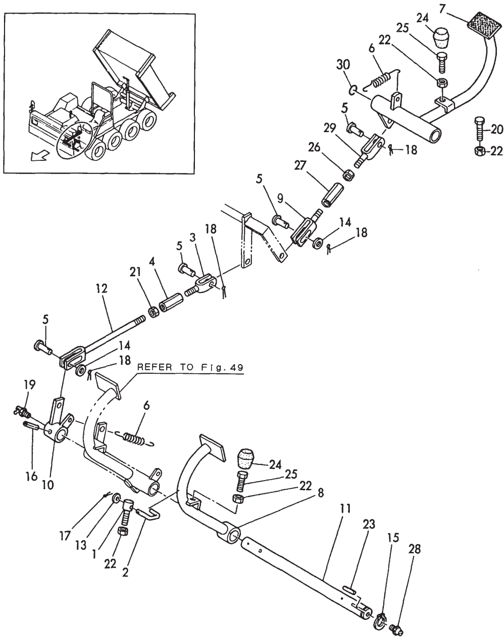
Fig.47 操縦装置 (クラッチペダル) CONTROL EQUIPMENT (CLUTCH PEDAL)
