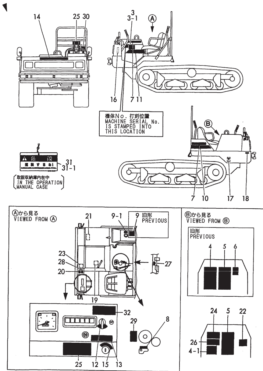
Fig. 10 銘板 (C30R-F) LABEL (C30R-F)
