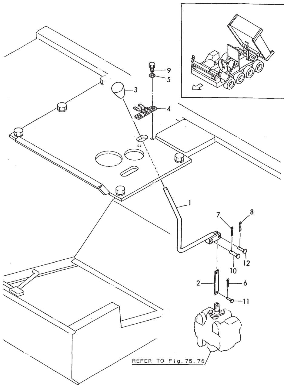
Fig. 51 油圧レバー HYD. OIL LEVER
