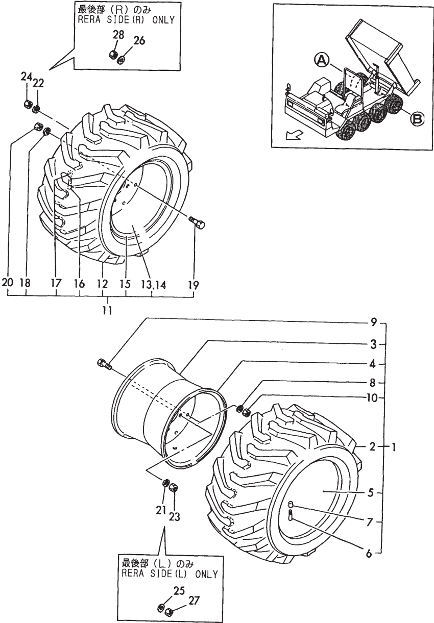
Fig.42 タイヤ&ホイール TIRE & WHEEL
