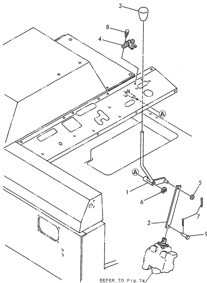
Fig. 50 油圧レバー (C20R) HYD. OIL LEVER (C20R)
