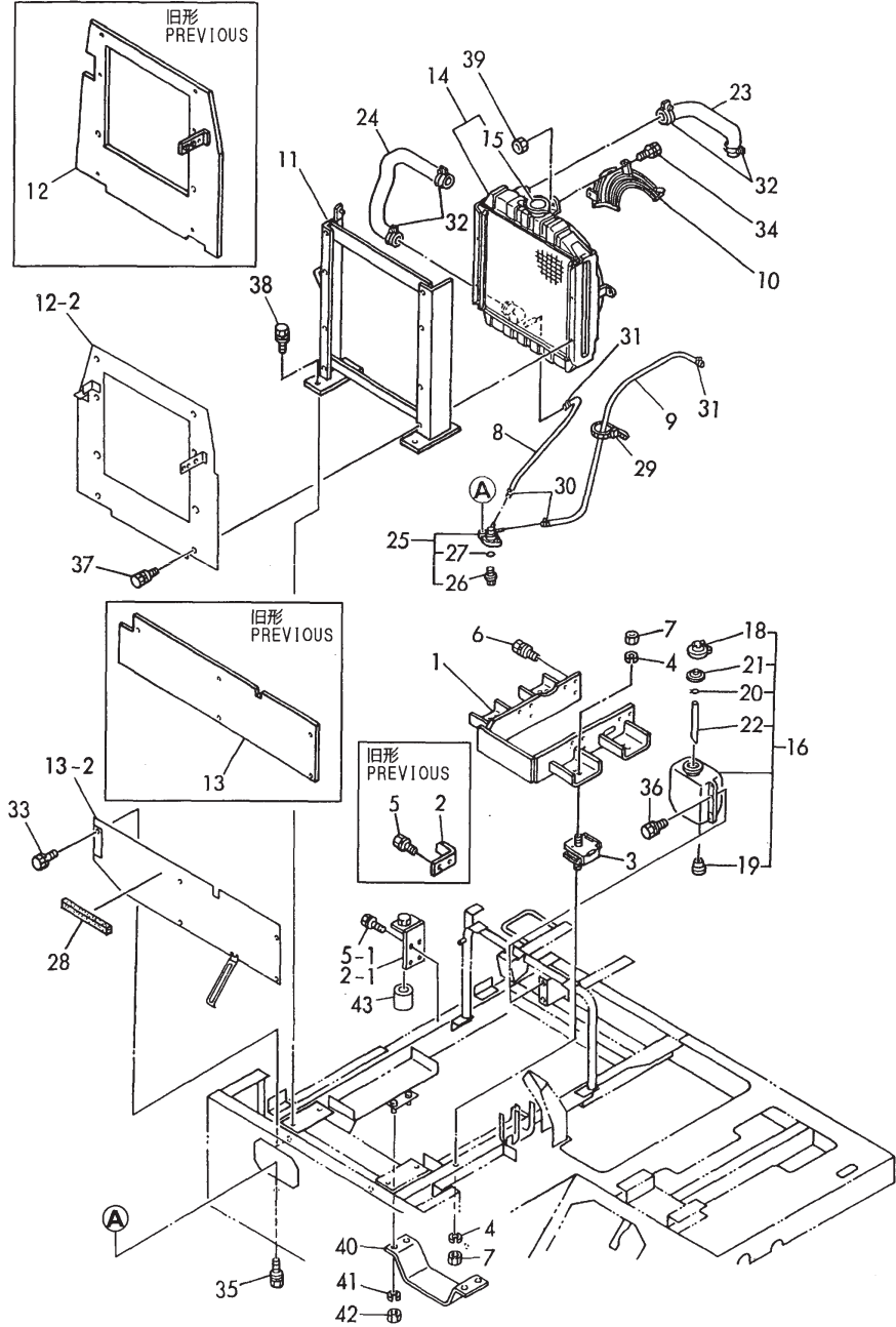
Fig. 18 エンジンマウント&ラジエータ (C20R) ENGINE MOUNT & RADIATOR (C20R)
