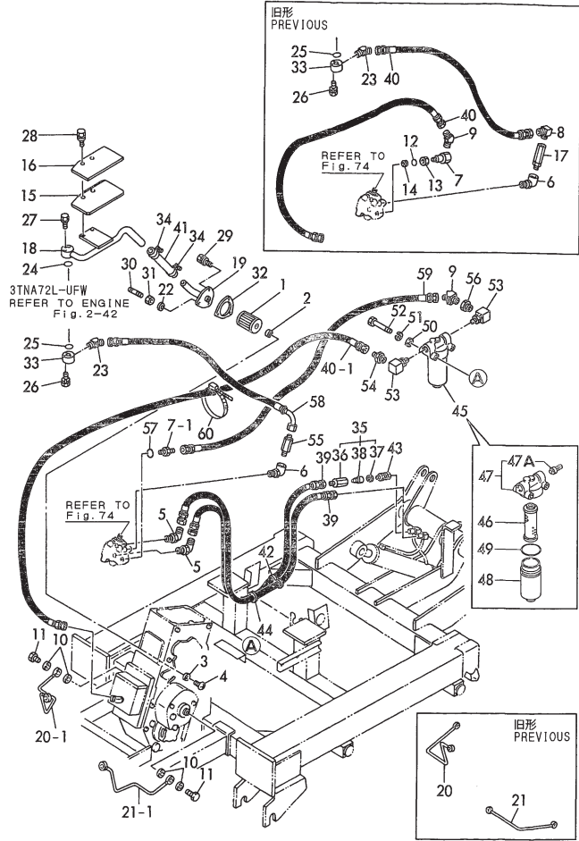
Fig. 66 油圧配管 (C20R) HYD.OIL PIPING (C20R)
