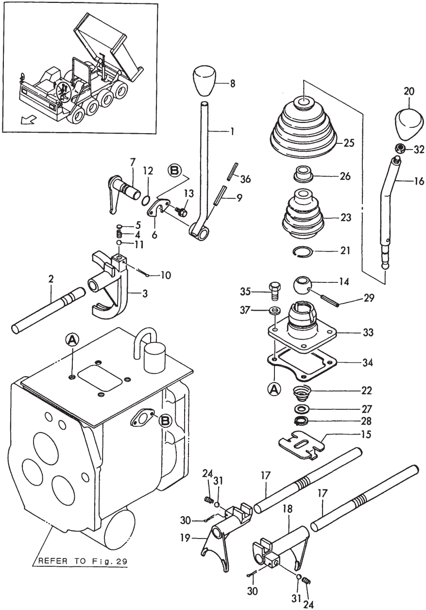
Fig.33 変速レバー SPEED CHANGE LEVER
