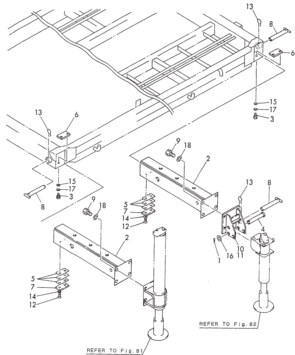
Fig.80 アウトリガマウント (C30R-2K) OUTRIGGER MOUNT (C30R-2K)
