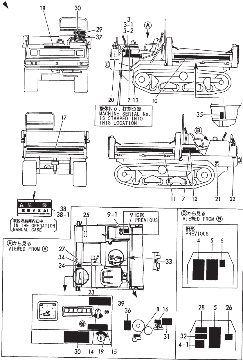
Fig.7 銘板 (C30R) (JP) LABEL (C30R) (JP)
