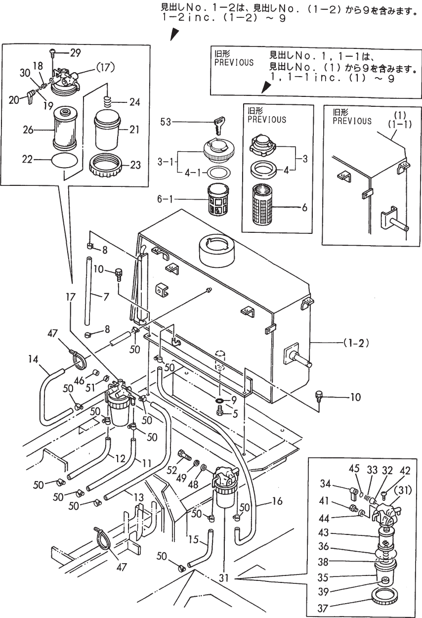
Fig.20 燃料タンク&燃料パイプ (C20R) FUEL TANK & FUEL LINE (C20R)
