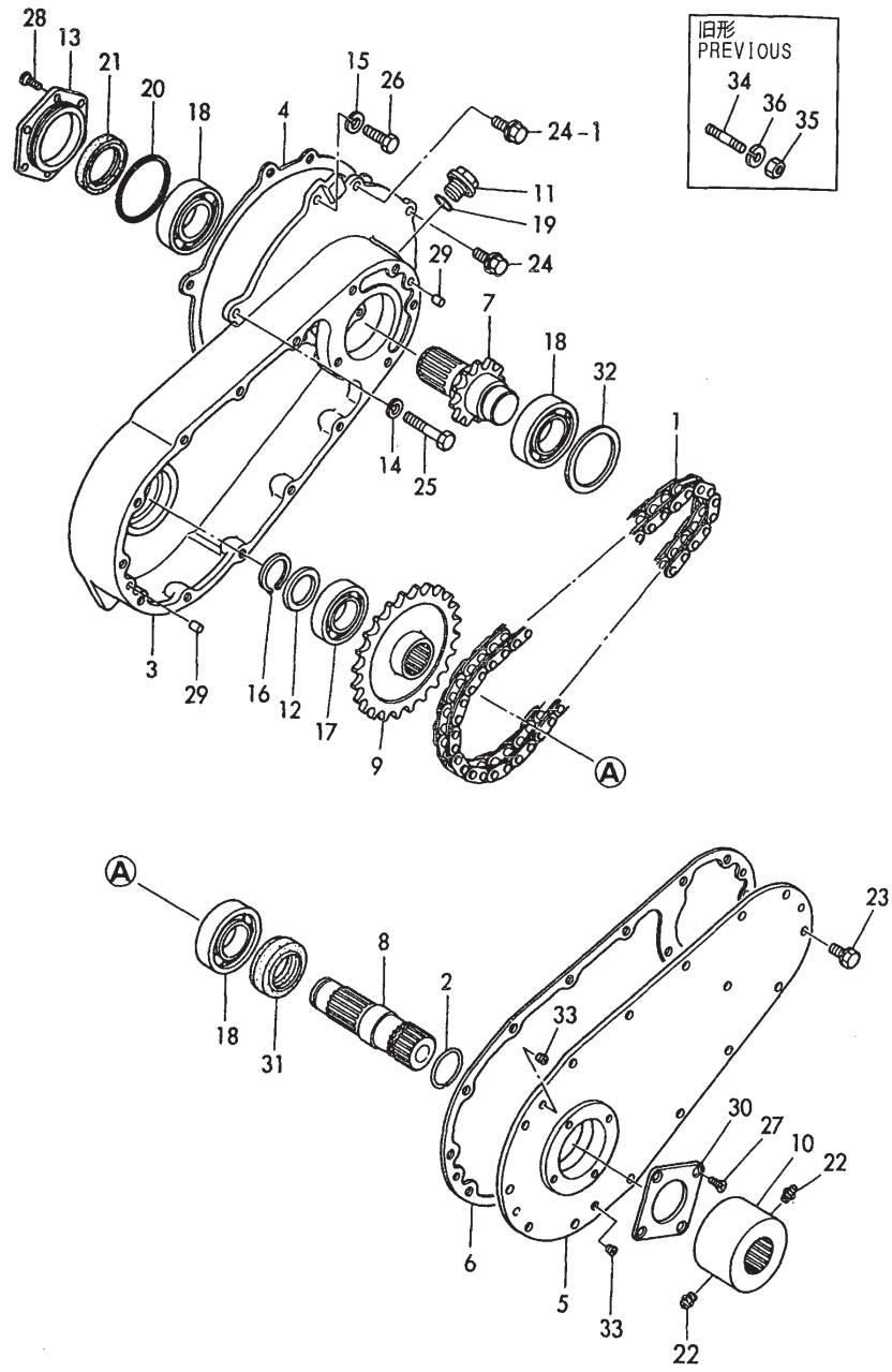
Fig.39 チェーンケース CHAIN CASE
