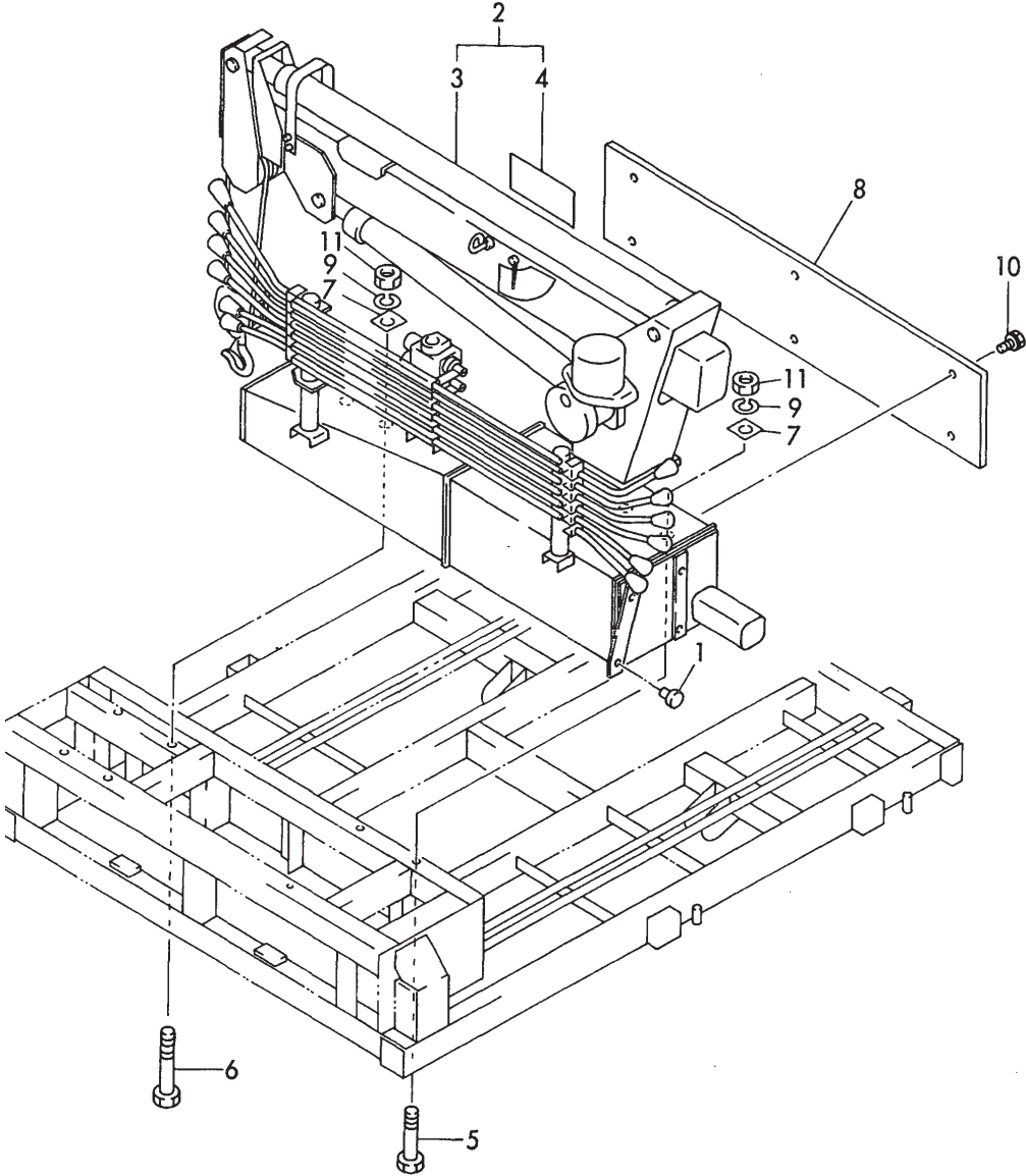
Fig.83 クレーン (C30R-1K) CRANE (C30R-1K)
