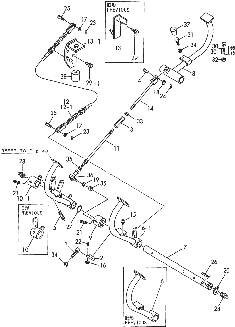
Fig.46 操縦装置 (クラッチペダル) (C20R) CONTROL EQUIPMENT (CLUTCH PEDAL) (C20R)
