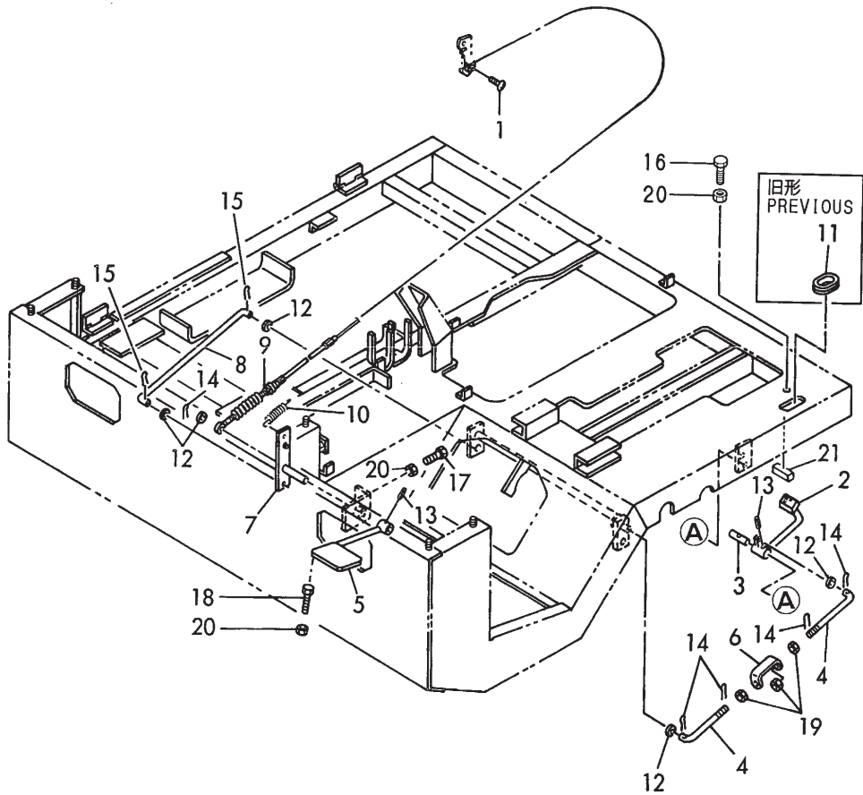
Fig. 16 フートアクセル (C20R) FOOT ACCELERATOR (C20R)
