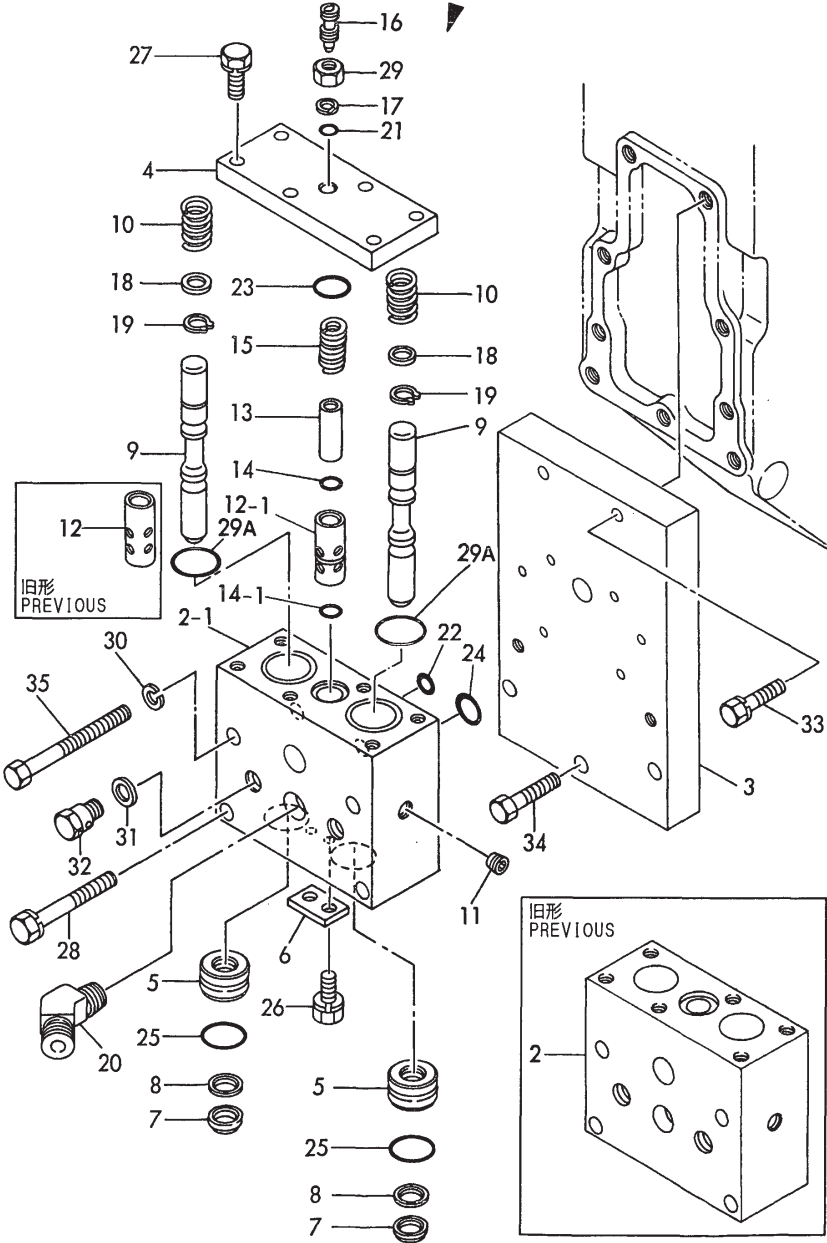
Fig.77 クラッチバルブ (C20R) CLUTCH VALVE (C20R)
