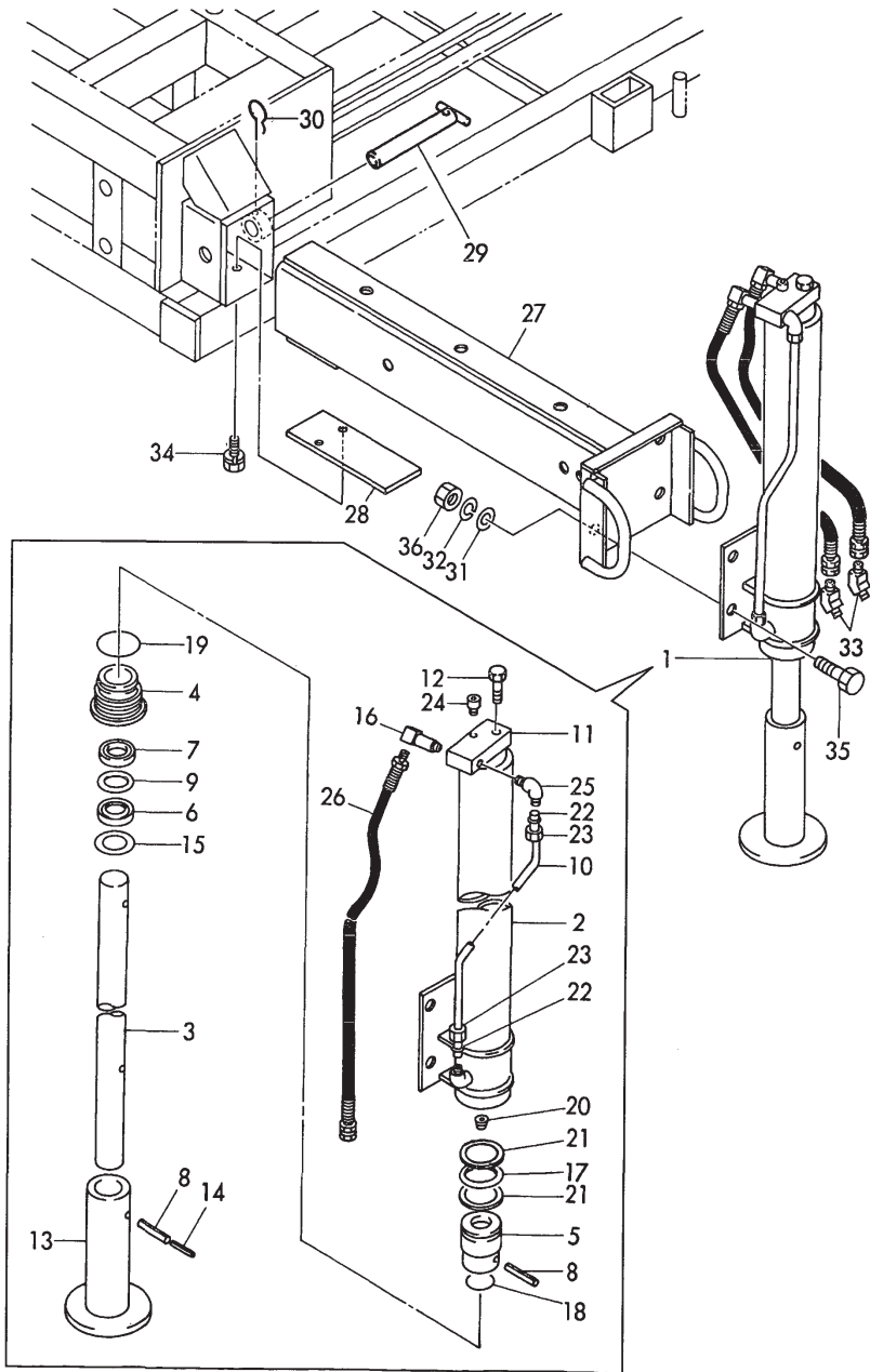
Fig. 79 アウトリガ (C30R-1K) OUTRIGGER (C30R-1K)
