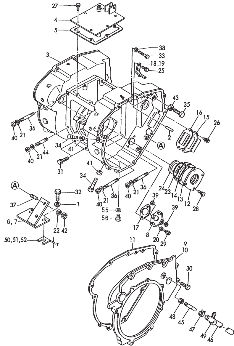
Fig.35 ステアリングケース (C30R) STEERING CASE (C30R)
