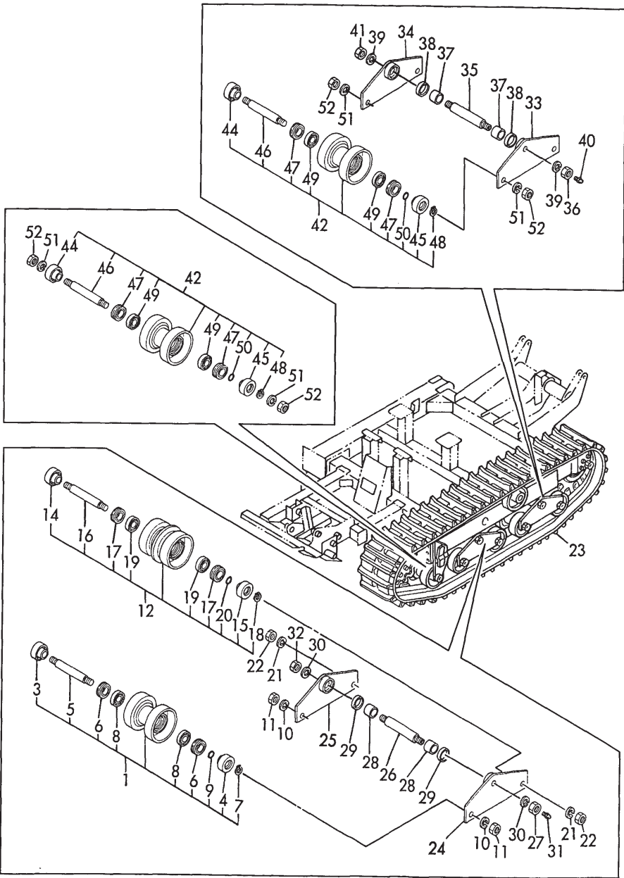
Fig.44 トラックローラ (C20R) TRACK ROLLER (C20R)
