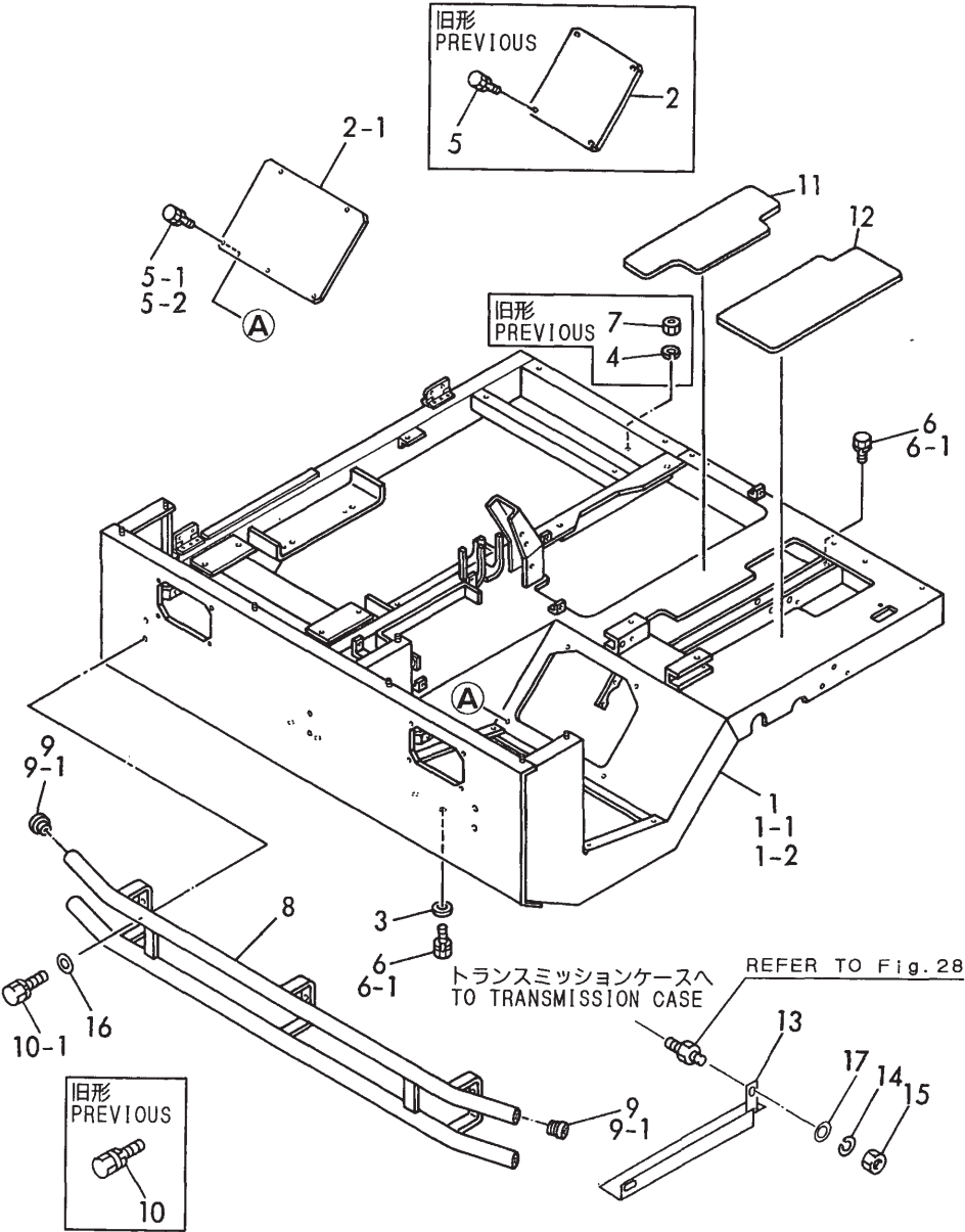
Fig.60 フロントフレーム (C20R) FRONT FRAME (C20R)
