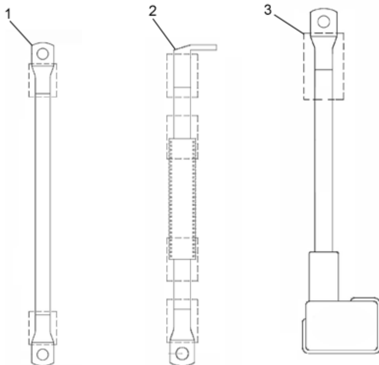
ESQUEMA CABLE MASA MASS CABLE DIAGRAM
