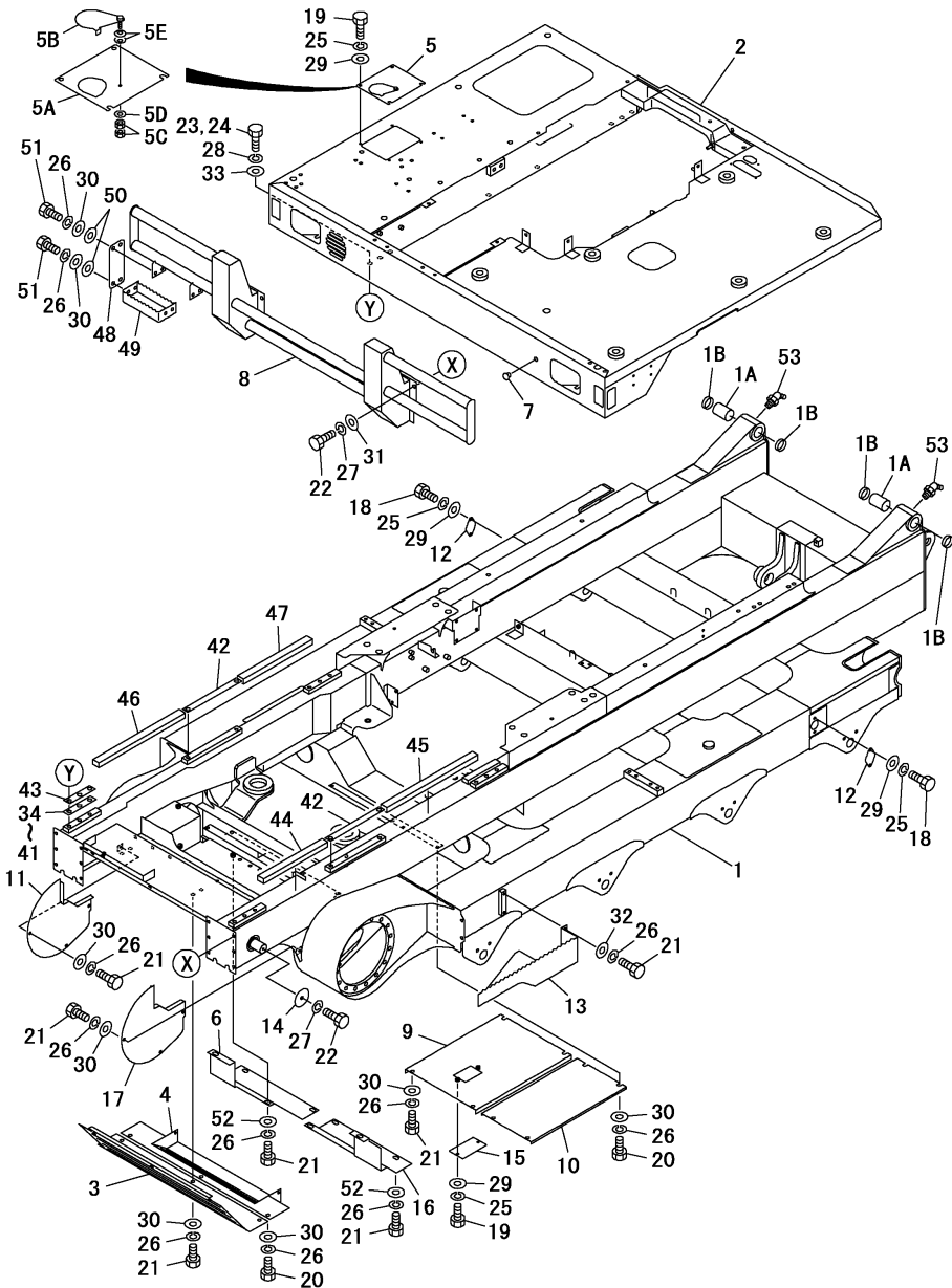
Fig.1. FRAME
