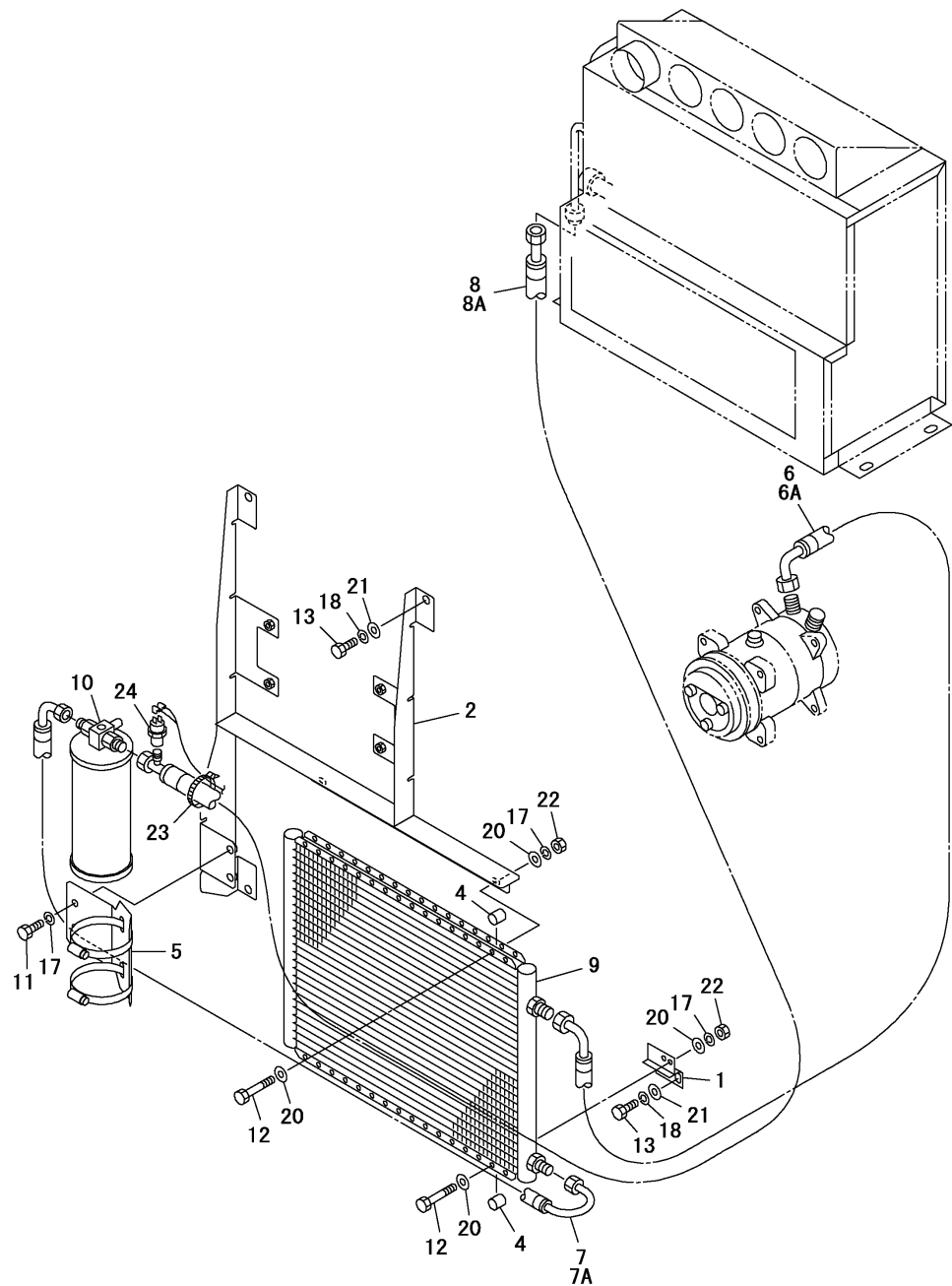
Fig.62. COOLER(2/5)(CONDENSER)
