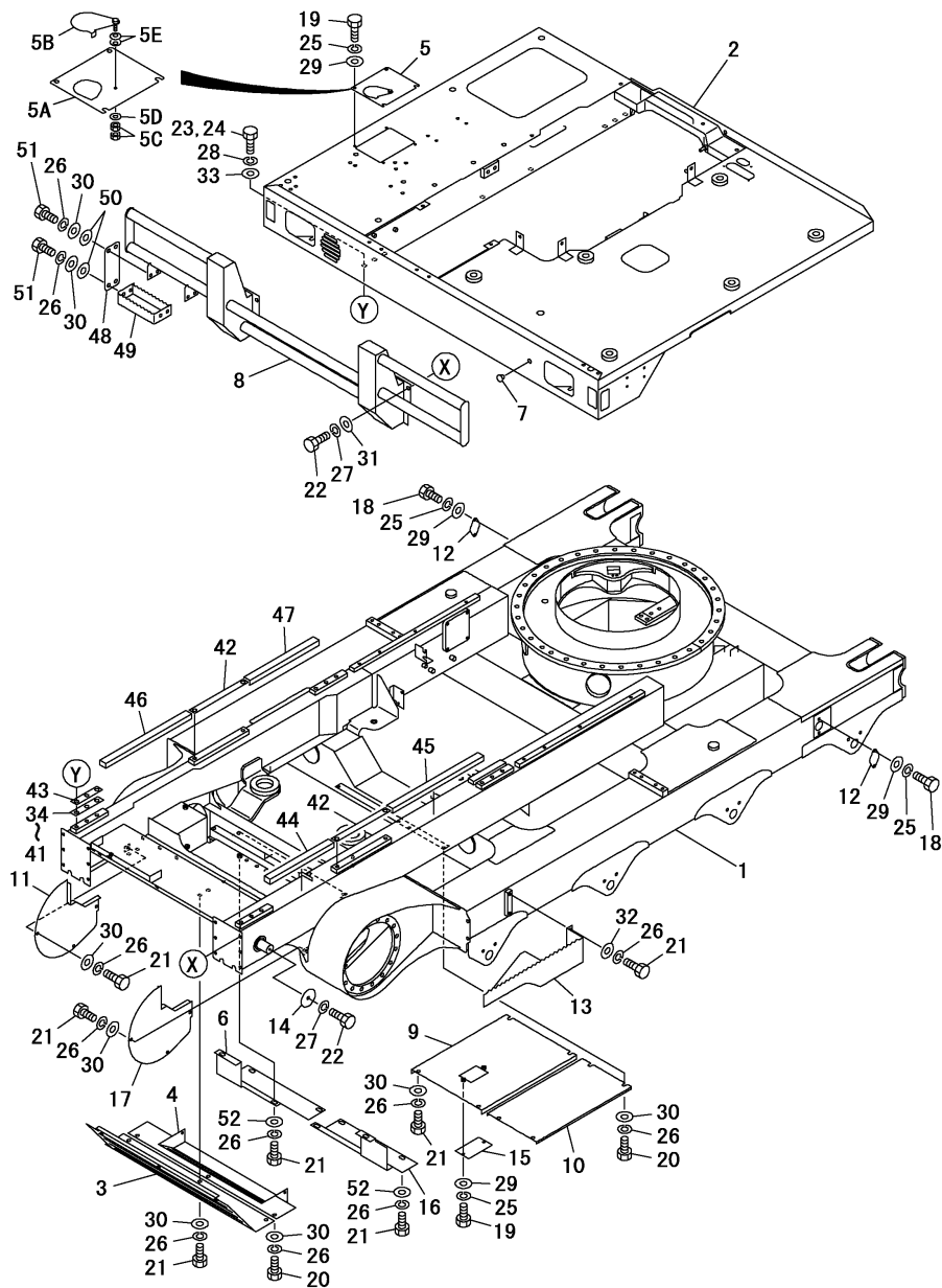
Fig.2. FRAME(TURNING)
