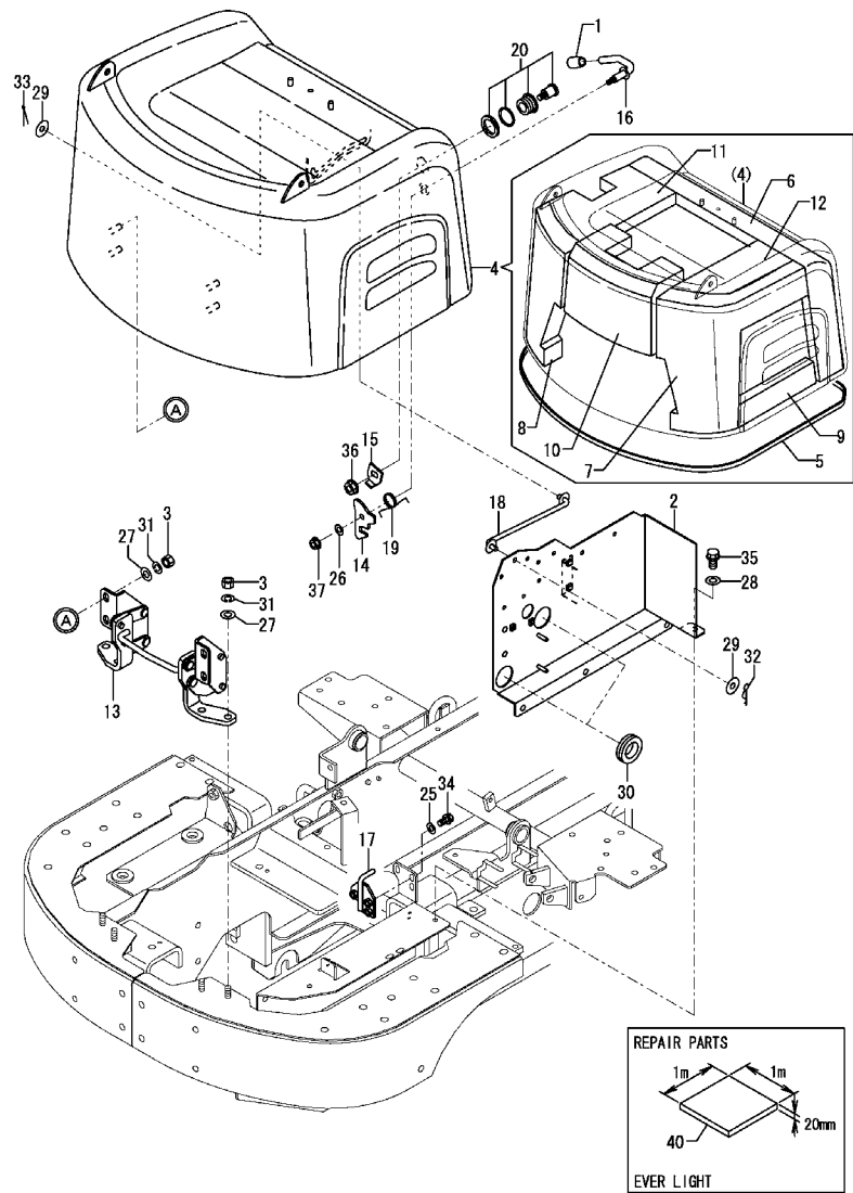
Fig.30. BONNET
