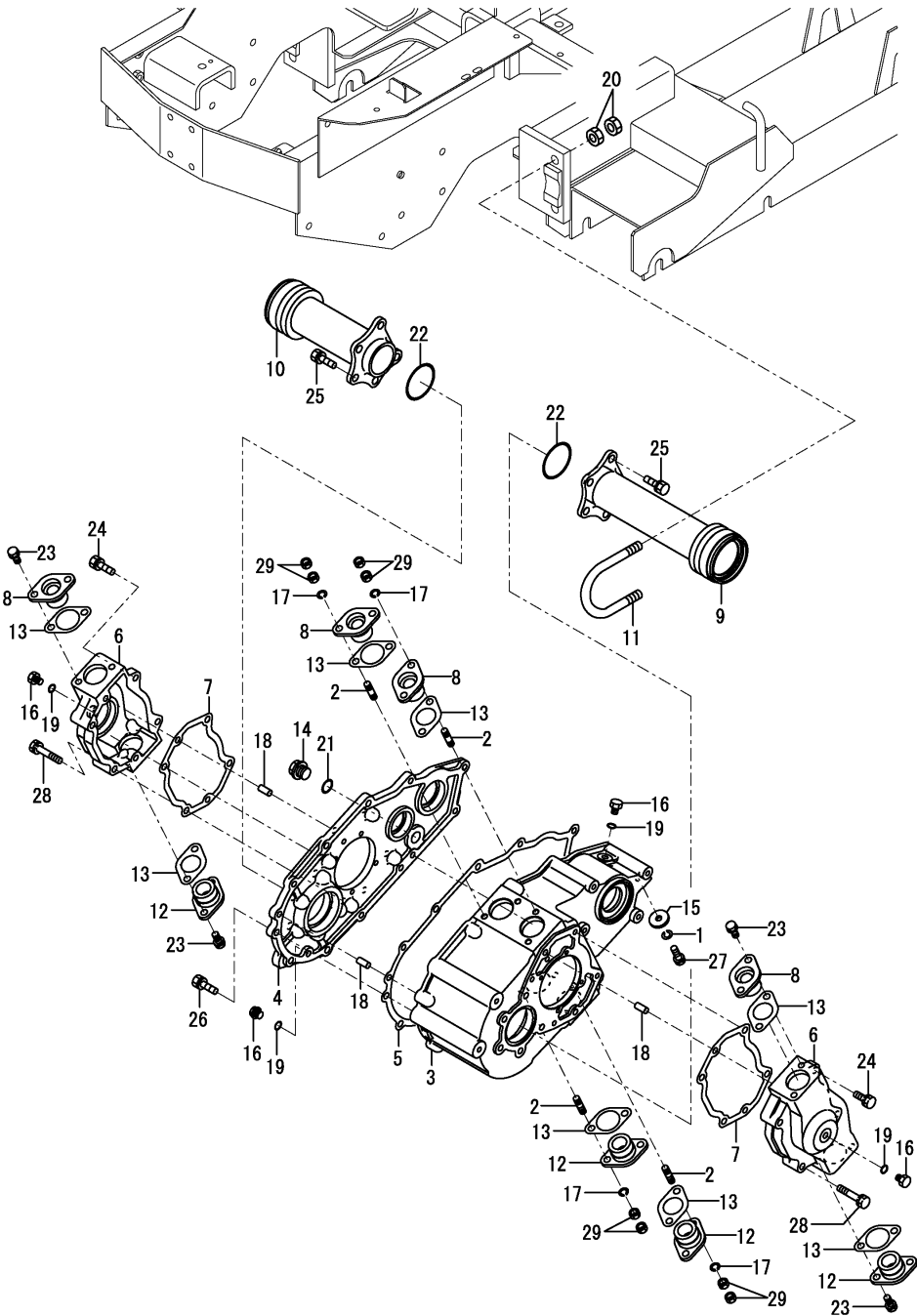
Fig.15. TRANSMISSION(CASE)
