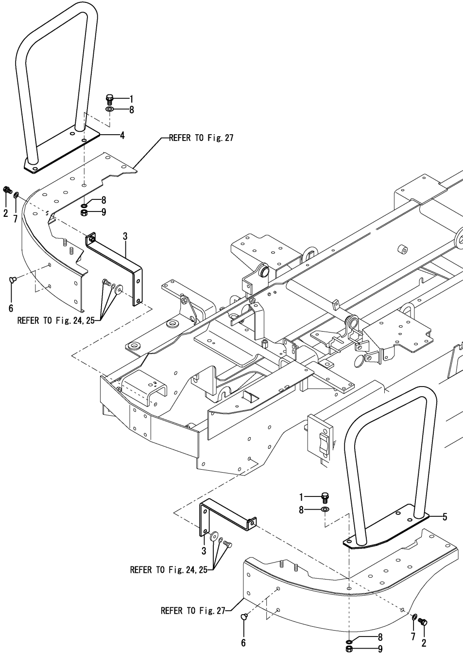
Fig.29. ASSIST BAR
