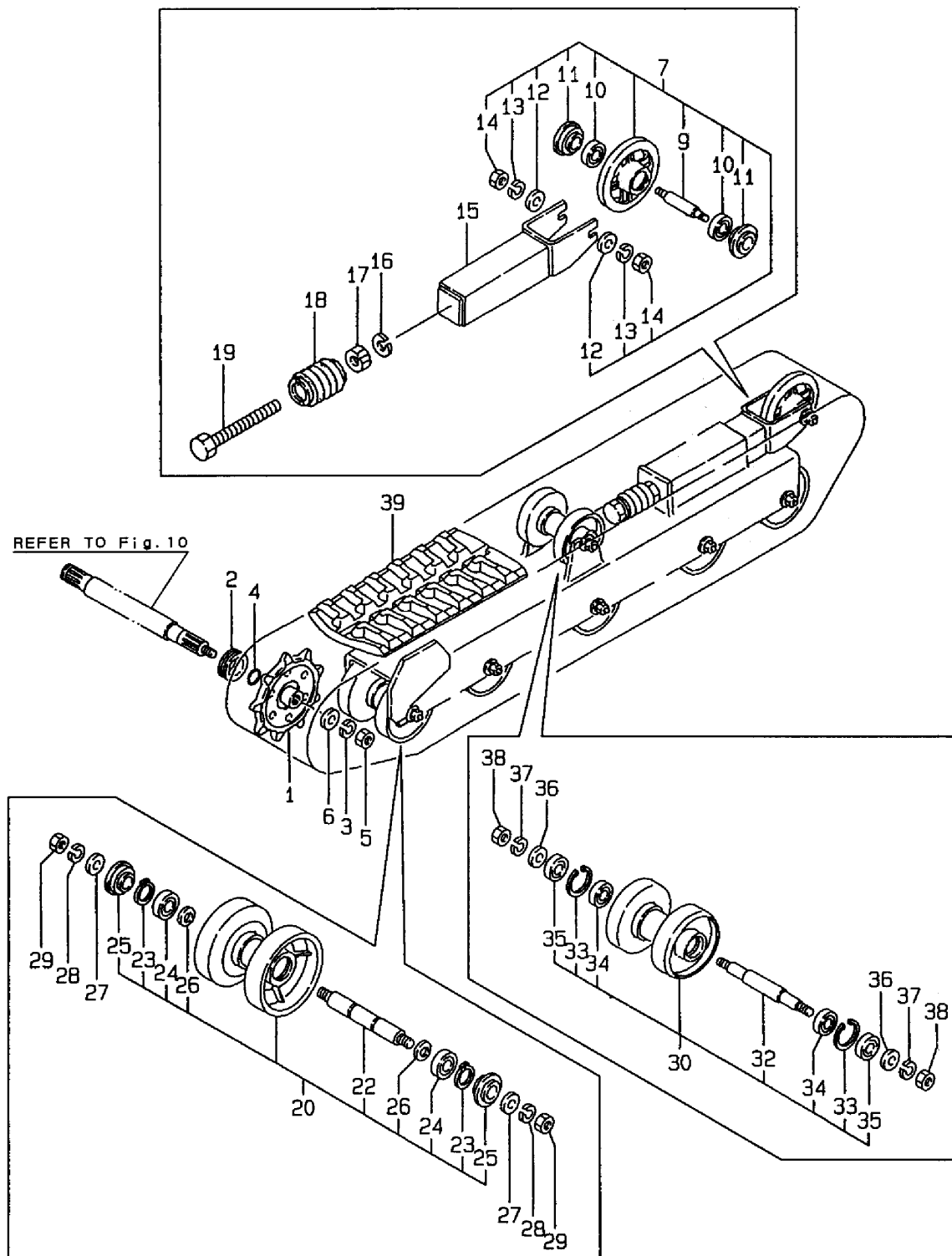
Fig. 13 クローラ関係 CRAWLER
