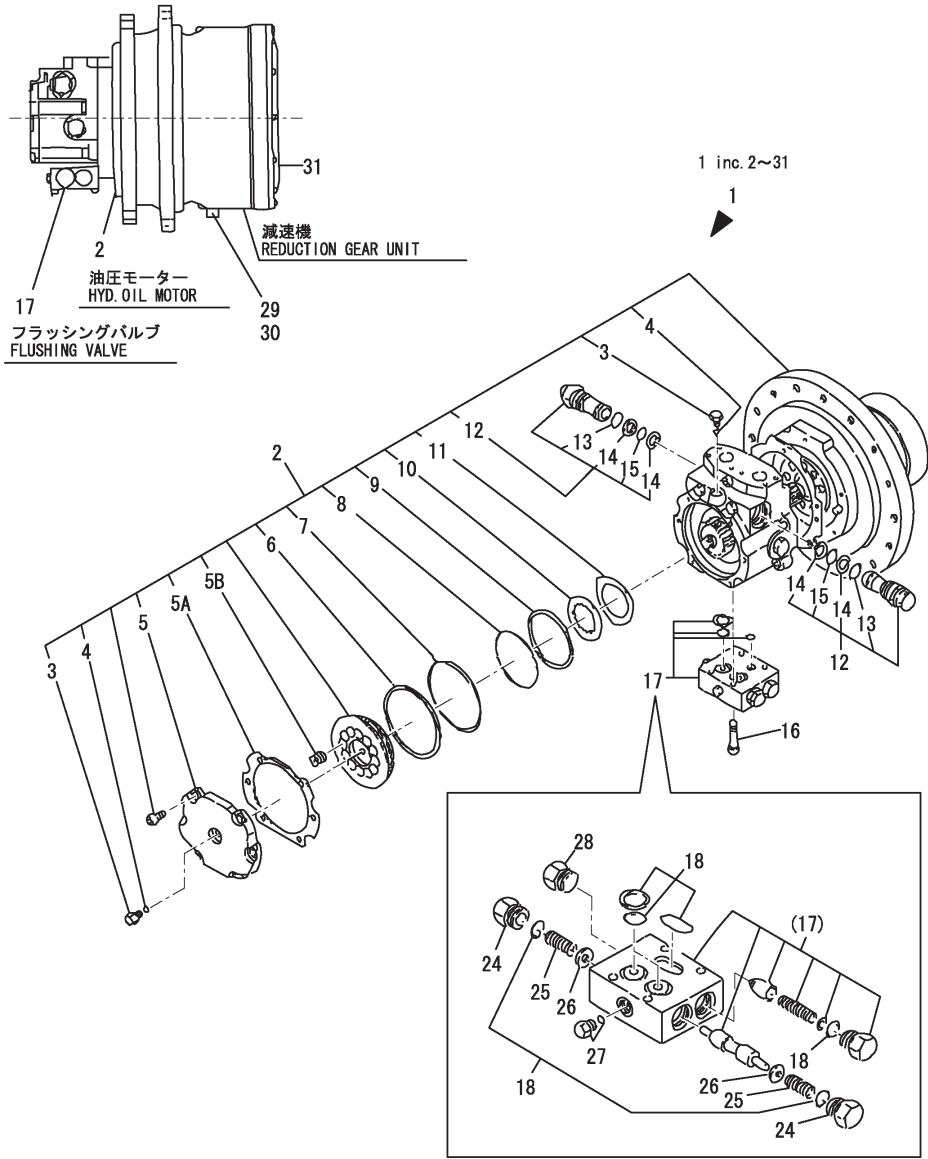
Fig.34. RUN MOTOR
