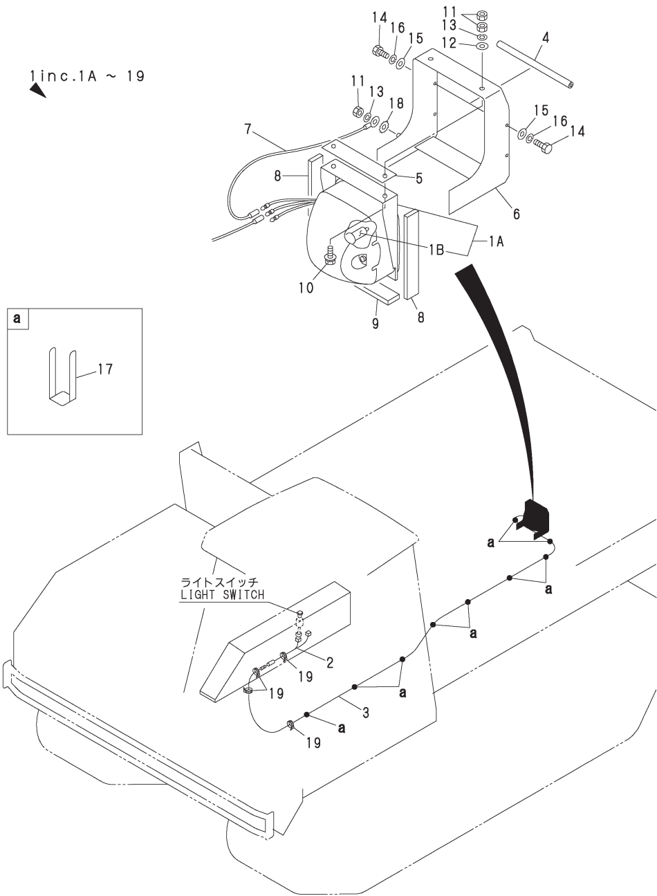
0CK30-G39501 Fig.41. TAIL LAMP
