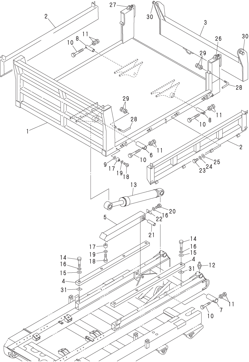
Fig.38. DUMP BODY
