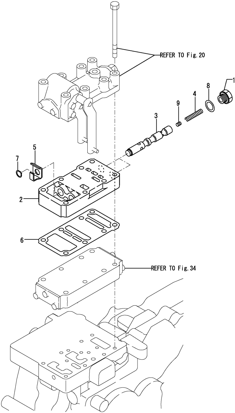
OCK30-G33302 Fig.33. SB VALVE
