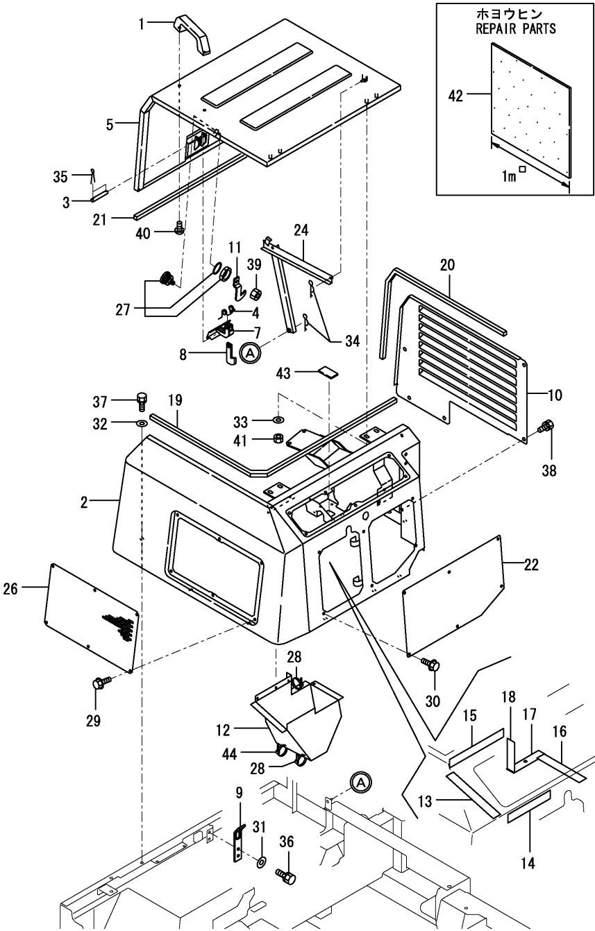
OCK30-G33302 Fig.39. BONNET
