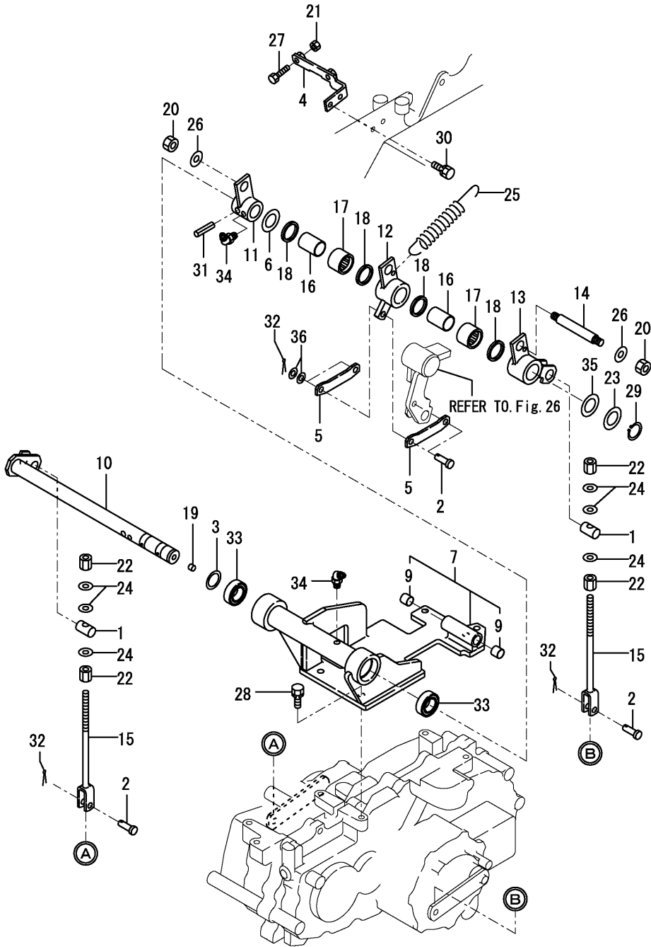
Fig.29. BRAKE(LINK)
