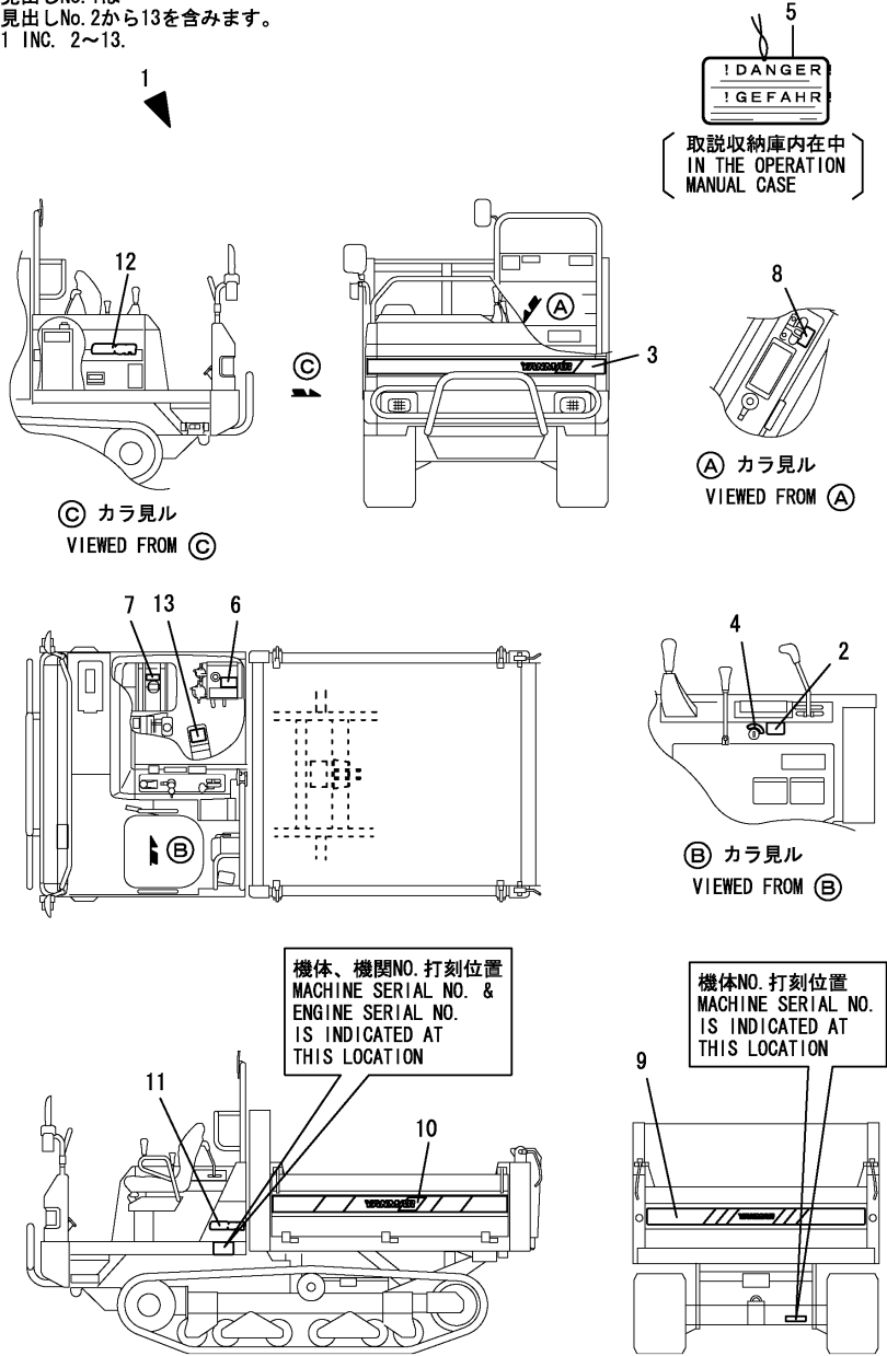
Fig.2. LABEL(EP)
